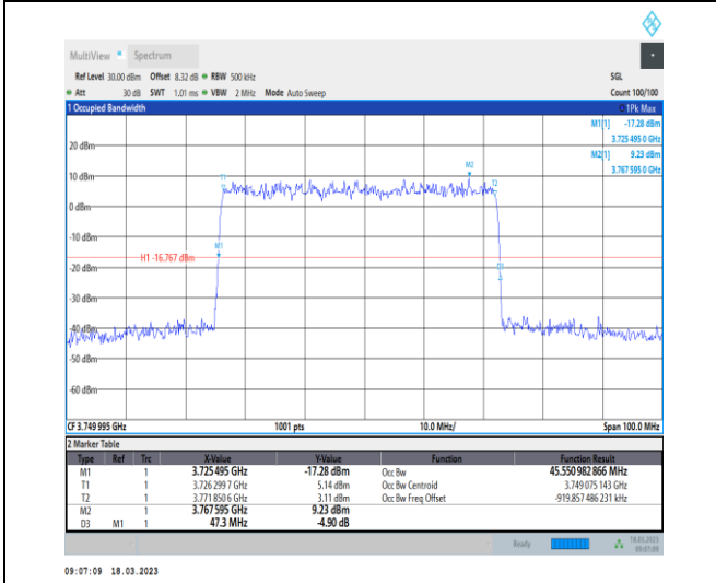
1-N78-3700-3800-30-50-M-5-DFT-256QAM-Outer_Full I-128@0-Ant0-45.551-47.300-≤50-PASS
