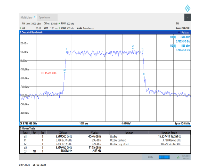
1-N78-3700-3800-30-20-H-1-DFT-QPSK-Outer_Full-50@0-Ant0-17.857-18.600-≤20-PASS
