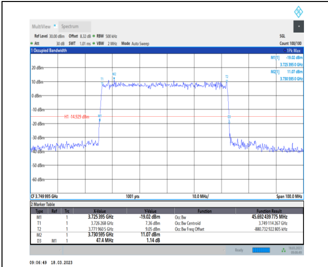
1-N78-3700-3800-30-50-M-3-DFT-16QAM-Outer_Ful I-128@0-Ant0-45.692-47.400-≤50-PASS
