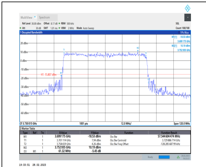
1-N78-3700-3800-30-60-L-5-DFT-256QAM-Outer_Fu II-162@0-Ant0-8.56-9.720-≤60-PASS
