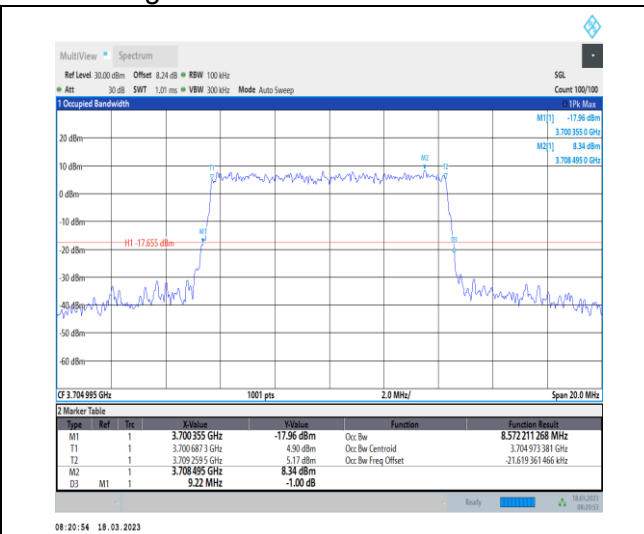
1-N78-3700-3800-30-10-L-6-CP-QPSK-Outer_Full-2 4@0-Ant0-8.572-9.220-≤10-PASS
