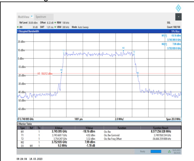
1-N78-3700-3800-30-10-M-5-DFT-256QAM-Outer_Full-24@0-Ant0-8.577-9.300-≤10-PASS
