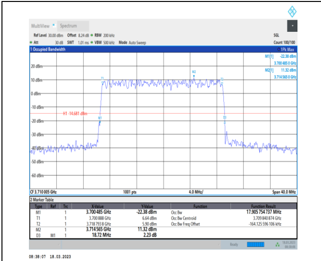
1-N78-3700-3800-30-20-L-3-DFT-16QAM-Outer_Full -50@0-Ant0-17.906-18.720-≤20-PASS
