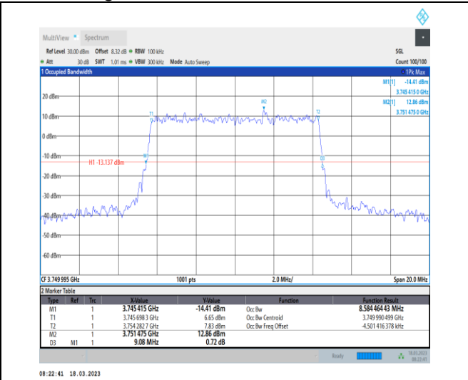
1-N78-3700-3800-30-10-M-1-DFT-QPSK-Outer_Full -24@0-Ant0-8.584-9.080-≤10-PASS
