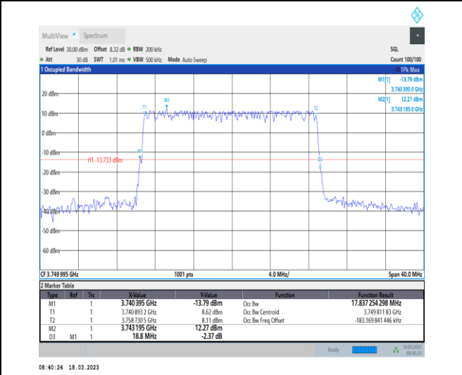
1-N78-3700-3800-30-20-M-1-DFT-QPSK-Outer_Full-50@0-Ant0-17.837-18.800-≤20-PASS
