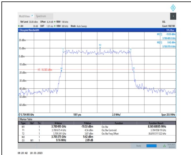
1-N78-3700-3800-30-10-L-5-DFT-256QAM-Outer_Fu II-24@0-Ant0-8.566-9.160-≤10-PASS
