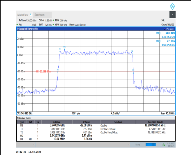
1-N78-3700-3800-30-20-M-9-CP-256QAM-Outer_Fu-51@0-Ant0-18.2-19.040-≤20-PASS
