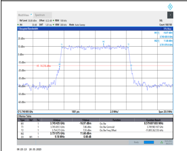
1-N78-3700-3800-30-10-M-2-DFT-PI2BPSK-Outer_F ull-24@0-Ant0-8.58-9.180-≤10-PASS
