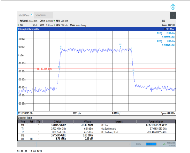
1-N78-3700-3800-30-20-L-5-DFT-256QAM-Outer_Fu II-50@0-Ant0-17.822-18.760-≤20-PASS
