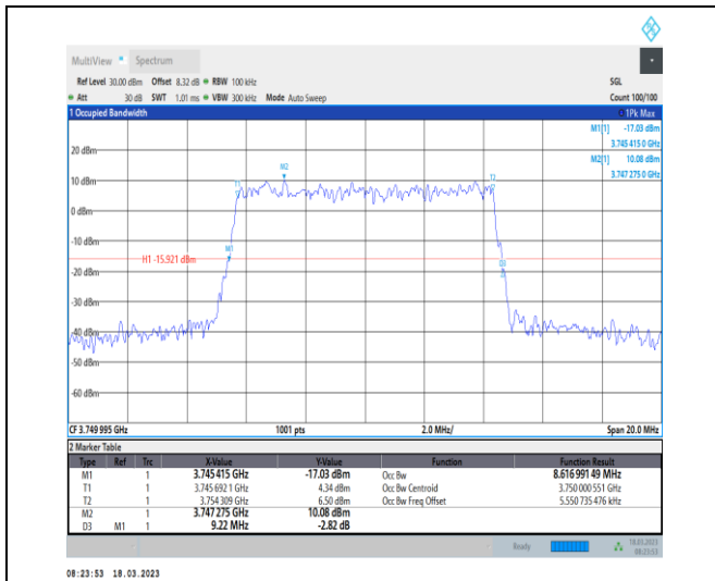
1-N78-3700-3800-30-10-M-4-DFT-64QAM-Outer_Ful I-24@0-Ant0-8.617-9.220-≤10-PASS
