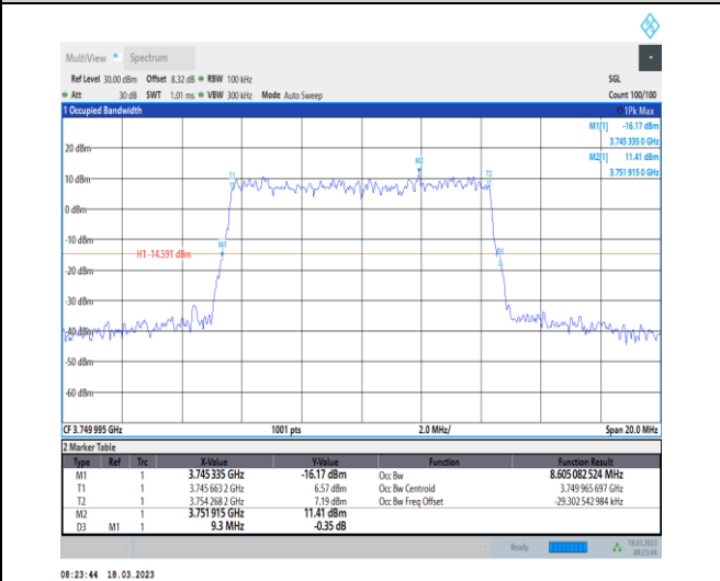
1-N78-3700-3800-30-10-M-3-DFT-16QAM-Outer_Ful l-24@0-Ant0-8.605-9.300-≤10-PASS
