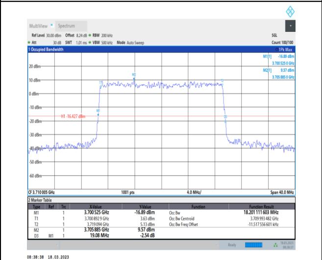
1-N78-3700-3800-30-20-L-6-CP-QPSK-Outer_Full-5 1@0-Ant0-18.201-19.080-≤20-PASS
