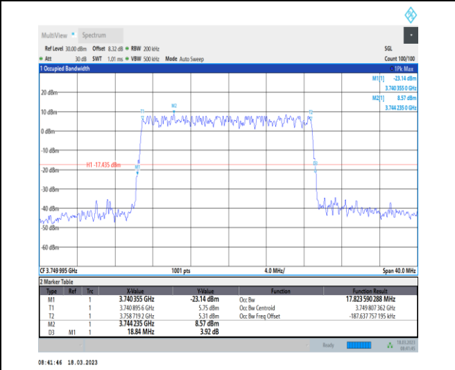
1-N78-3700-3800-30-20-M-5-DFT-256QAM-Outer_Full-50@0-Ant0-17.824-18.840-≤20-PASS
