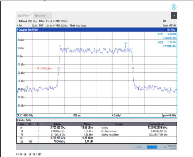
1-N78-3700-3800-30-20-L-4-DFT-64QAM-Outer_Full -50@0-Ant0-17.799-18.560-≤20-PASS
