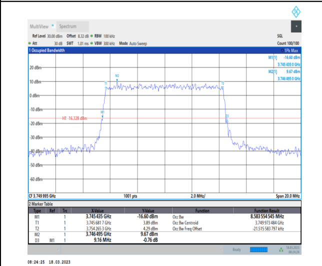
1-N78-3700-3800-30-10-M-7-CP-16QAM-Outer_Full-24@0-Ant0-8.584-9.160-≤10-PASS
