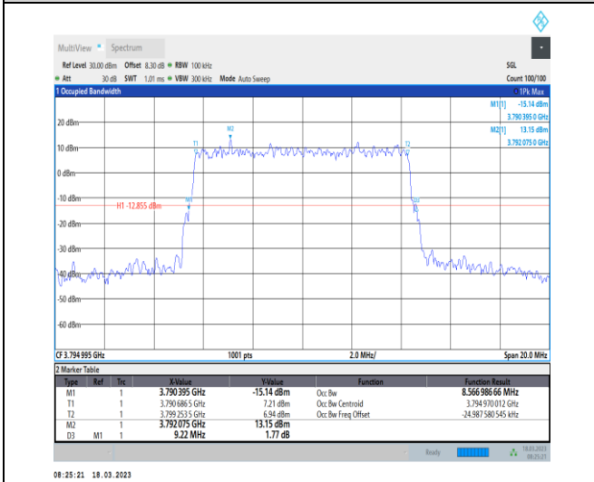
1-N78-3700-3800-30-10-H-1-DFT-QPSK-Outer_Full-24@0-Ant0-8.567-9.220-≤10-PASS
