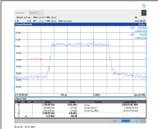
1-N78-3700-3800-30-10-L-9-CP-256QAM-Outer_Full -24@0-Ant0-8.595-9.140-≤10-PASS
