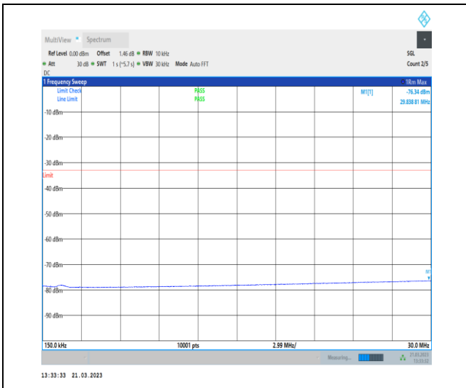
1-N78-3450-3550-30-100-M-1-DFT-QPSK-Edge_1R B_Left-1@0-0.15-30-Ant0-29.84--76.34--33-PASS
