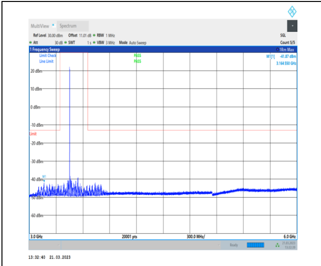
1-N78-3450-3550-30-100-L-1-DFT-QPSK-Edge_1R B_Left-1@0-3000-6000-Ant0-3164.55--41.87--13-PA SS
