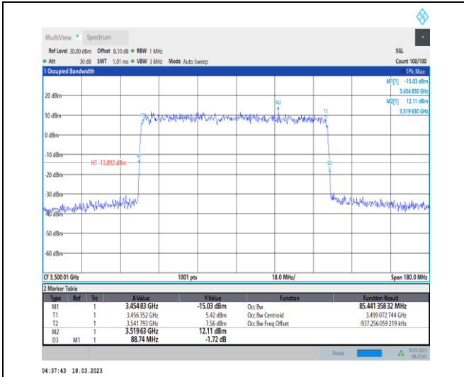
1-N78-3450-3550-30-90-M-3-DFT-16QAM-Outer_Ful I-240@0-Ant0-85.441-88.740-≤90-PASS
