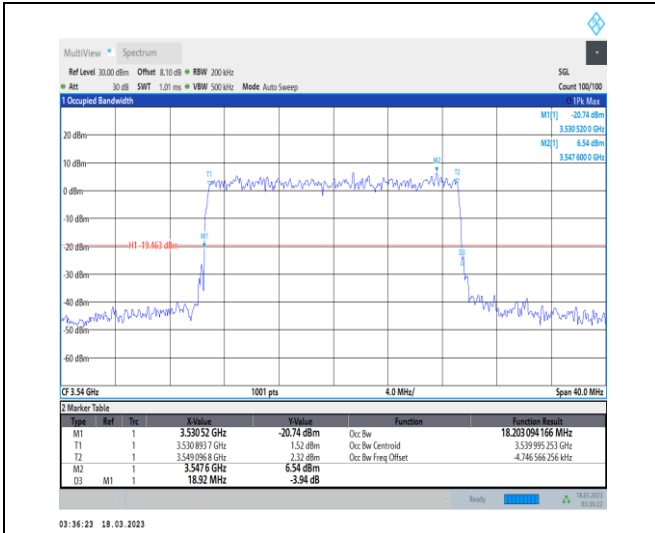
1-N78-3450-3550-30-20-H-9-CP-256QAM-Outer_Ful I-51@0-Ant0-18.203-18.920-≤20-PASS
