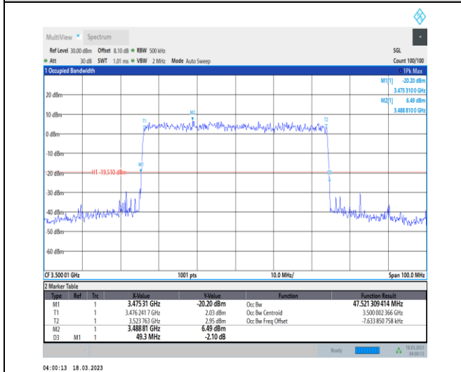
1-N78-3450-3550-30-50-M-9-CP-256QAM-Outer_Ful-133@0-Ant0-47.521-49.300-≤50-PASS
