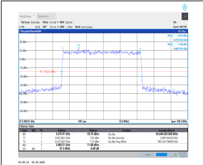
1-N78-3450-3550-30-50-M-3-DFT-16QAM-Outer_Ful I-128@0-Ant0-45.644-47.500-≤50-PASS
