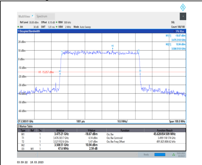
1-N78-3450-3550-30-50-M-4-DFT-64QAM-Outer_Ful I-128@0-Ant0-45.629-47.600-≤50-PASS
