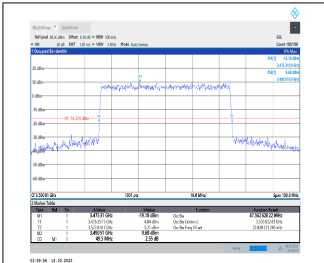
1-N78-3450-3550-30-50-M-7-CP-16QAM-Outer_Full-133@0-Ant0-47.563-49.500-≤50-PASS
