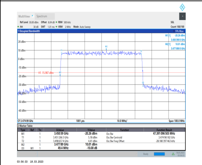
1-N78-3450-3550-30-50-L-7-CP-16QAM-Outer_Full-133@0-Ant0-47.391-49.400-≤50-PASS
