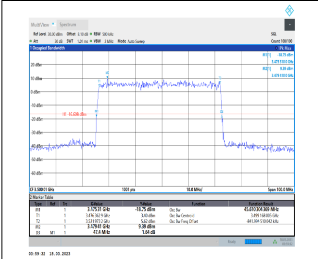
1-N78-3450-3550-30-50-M-5-DFT-256QAM-Outer_Full-128@0-Ant0-45.61-47.400-≤50-PASS
