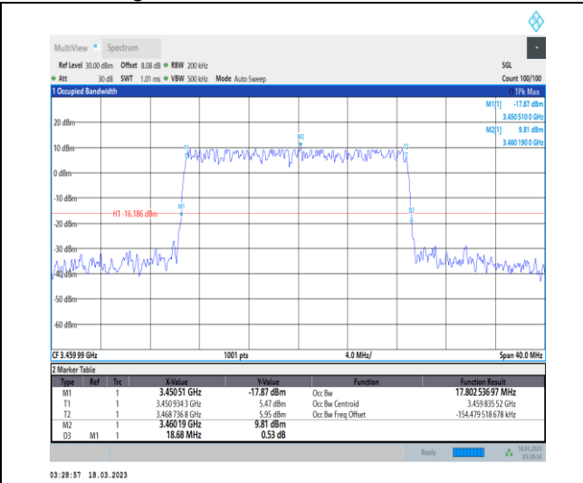
1-N78-3450-3550-30-20-L-4-DFT-64QAM-Outer_Full -50@0-Ant0-17.803-18.680-≤20-PASS
