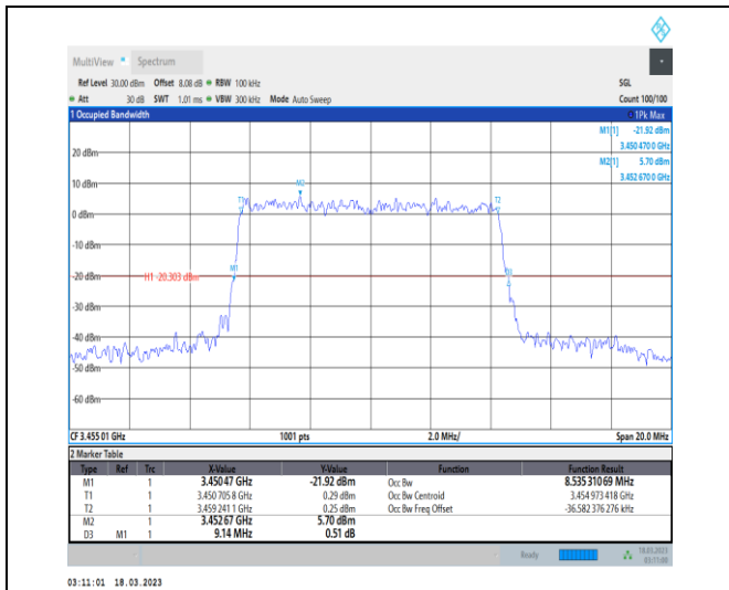
1-N78-3450-3550-30-10-L-9-CP-256QAM-Outer_Full -24@0-Ant0-8.535-9.140-≤10-PASS
