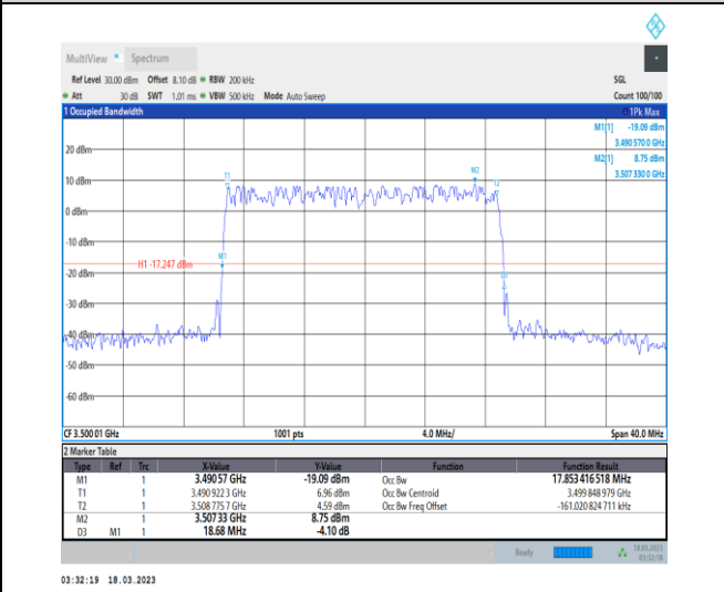
1-N78-3450-3550-30-20-M-5-DFT-256QAM-Outer_Full-50@0-Ant0-17.853-18.680-≤20-PASS
