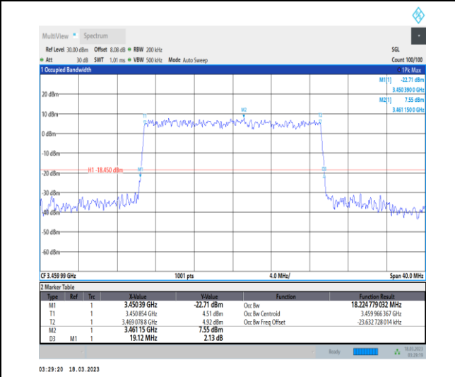
1-N78-3450-3550-30-20-L-6-CP-QPSK-Outer_Full-5 1@0-Ant0-18.225-19.120-≤20-PASS
