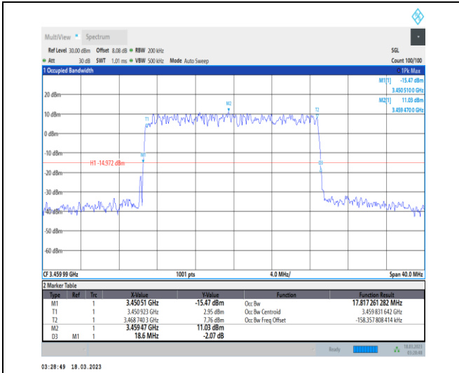
1-N78-3450-3550-30-20-L-3-DFT-16QAM-Outer_Full -50@0-Ant0-17.817-18.600-≤20-PASS
