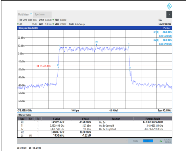
1-N78-3450-3550-30-20-L-5-DFT-256QAM-Outer_Fu II-50@0-Ant0-17.839-18.520-≤20-PASS
