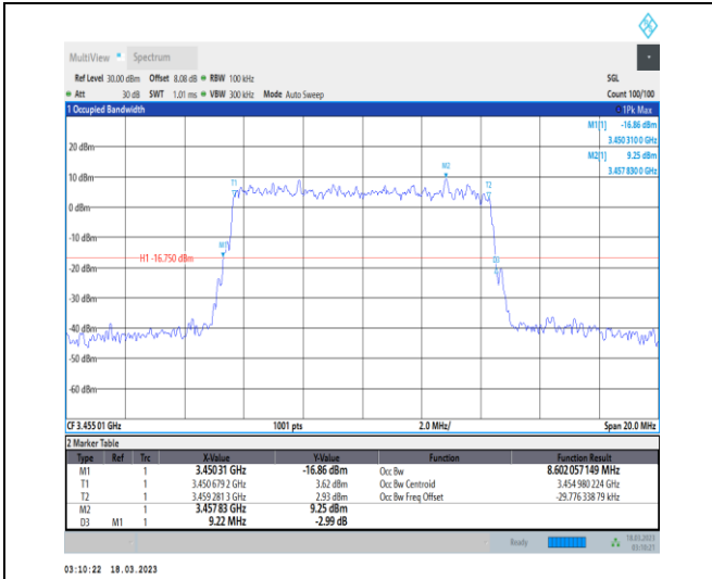
1-N78-3450-3550-30-10-L-5-DFT-256QAM-Outer_Fu II-24@0-Ant0-8.602-9.220-≤10-PASS
