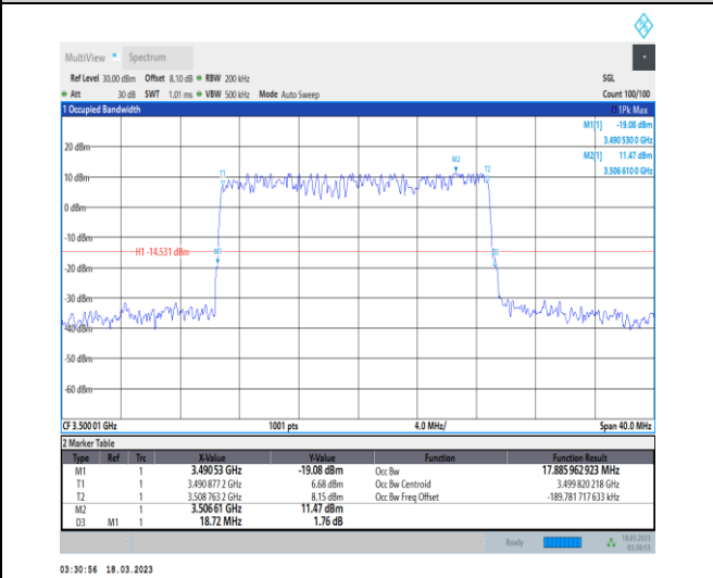
1-N78-3450-3550-30-20-M-1-DFT-QPSK-Outer_Full-50@0-Ant0-17.886-18.720-≤20-PASS
