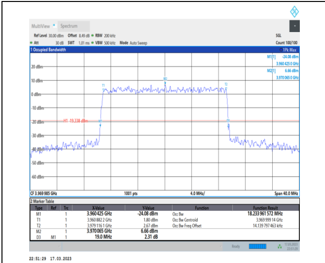
1-N77-3700-3980-30-20-H-9-CP-256QAM-Outer_Ful I-51@0-Ant0-18.234-19.000-≤20-PASS
