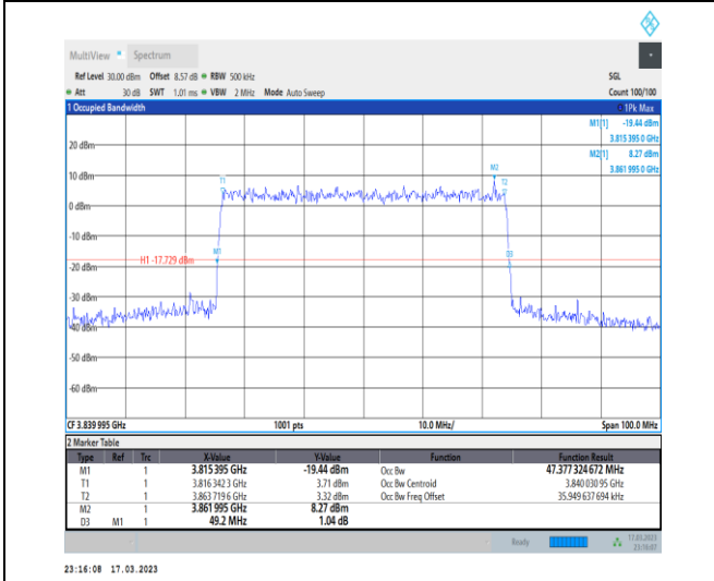
1-N77-3700-3980-30-50-M-9-CP-256QAM-Outer_Ful-I-133@0-Ant0-47.377-49.200-≤50-PASS
