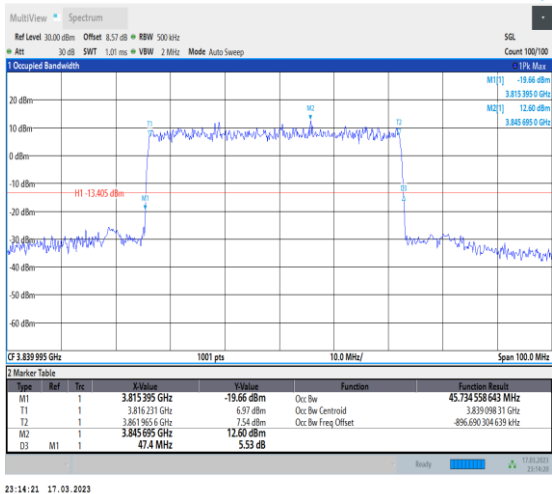
1-N77-3700-3980-30-50-M-3-DFT-16QAM-Outer_Ful I-128@0-Ant0-45.735-47.400-≤50-PASS
