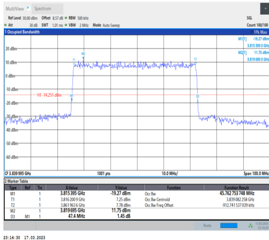
1-N77-3700-3980-30-50-M-4-DFT-64QAM-Outer_Ful I-128@0-Ant0-45.763-47.400-≤50-PASS
