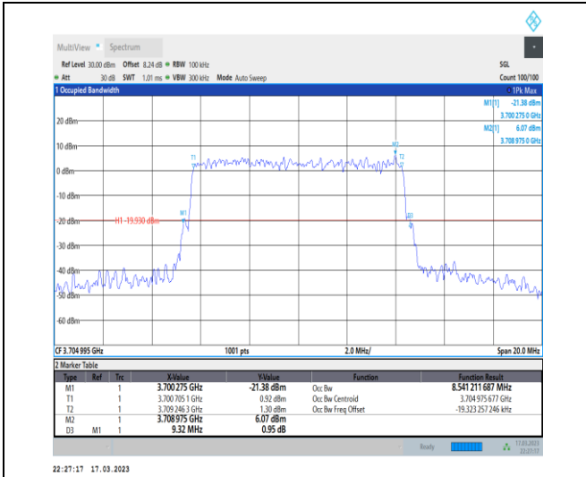
1-N77-3700-3980-30-10-L-9-CP-256QAM-Outer_Full -24@0-Ant0-8.541-9.320-≤10-PASS
