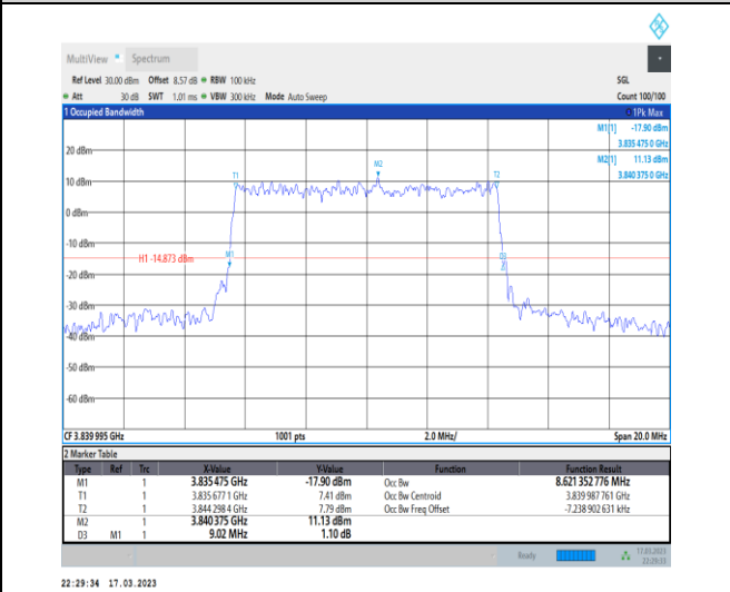
1-N77-3700-3980-30-10-M-3-DFT-16QAM-Outer_Ful l-24@0-Ant0-8.621-9.020-≤10-PASS
