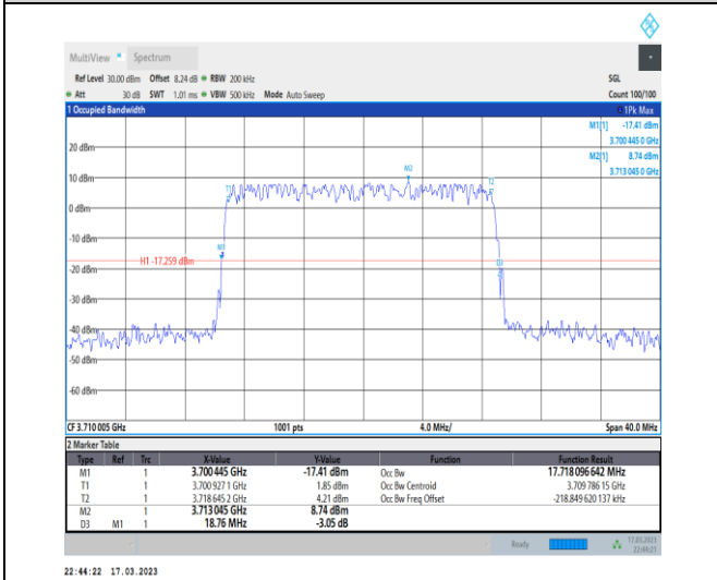
1-N77-3700-3980-30-20-L-5-DFT-256QAM-Outer_Fu II-50@0-Ant0-17.718-18.760-≤20-PASS
