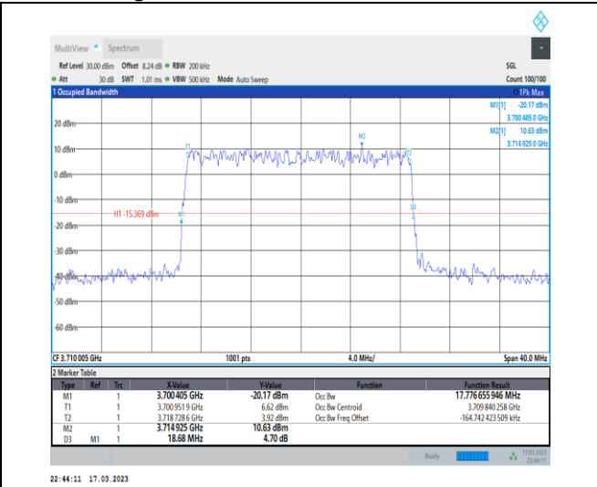
1-N77-3700-3980-30-20-L-4-DFT-64QAM-Outer_Full -50@0-Ant0-17.777-18.680-≤20-PASS
