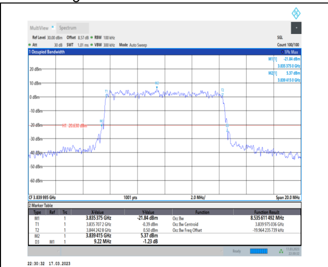
1-N77-3700-3980-30-10-M-9-CP-256QAM-Outer_FuII-24@0-Ant0-8.536-9.220-≤10-PASS
