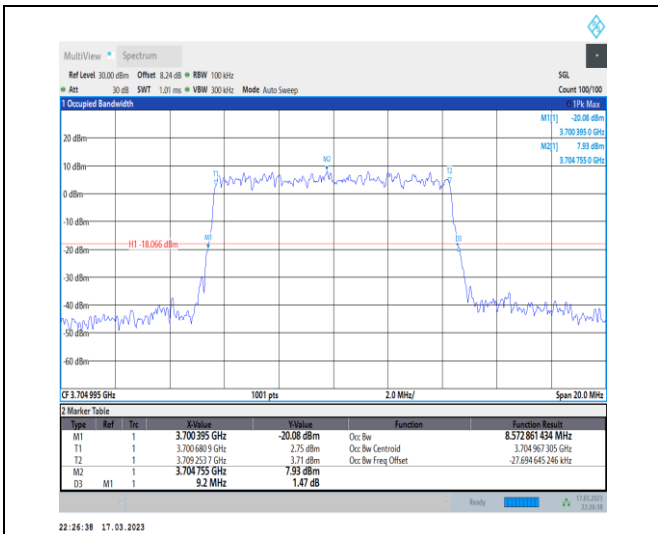
1-N77-3700-3980-30-10-L-5-DFT-256QAM-Outer_Fu II-24@0-Ant0-8.573-9.200-≤10-PASS
