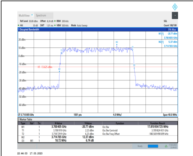
1-N77-3700-3980-30-20-L-3-DFT-16QAM-Outer_Full -50@0-Ant0-17.811-18.720-≤20-PASS
