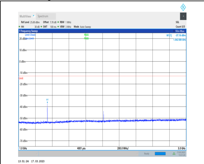
1-N71-PC3-15-20-M-1-DFT-PI2BPSK-Inner_1RB_L eft-1@1-1000-3000-Ant7-1342.50--37.16--13-PASS
