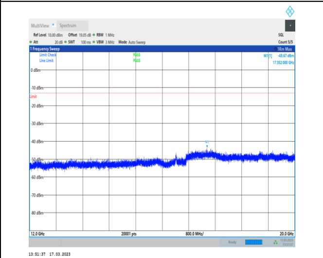
1-N71-PC3-15-20-M-1-DFT-PI2BPSK-Inner_1RB_L eft-1@1-12000-20000-Ant7-17352.00--43.67--13-PASS
