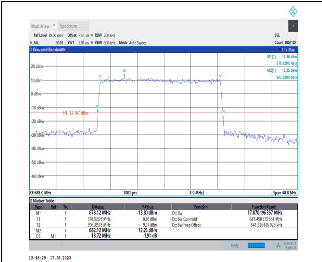
1-N71-PC3-15-20-H-3-DFT-16QAM-Outer_Full-100 @0-Ant7-17.87-18.720-≤20-PASS
