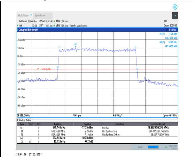
1-N71-PC3-15-20-H-8-CP-64QAM-Outer_Full-106@ 0-Ant7-18.894-19.720-≤20-PASS
