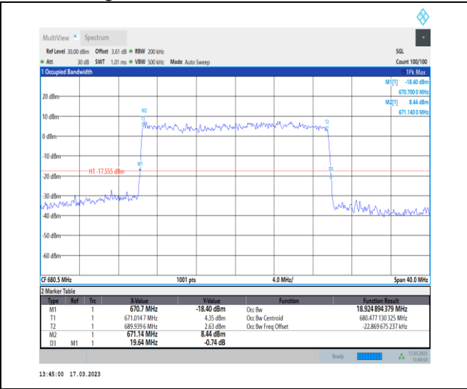
1-N71-PC3-15-20-M-9-CP-256QAM-Outer_Full-106 @0-Ant7-18.925-19.640-≤20-PASS
