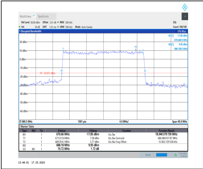
1-N71-PC3-15-20-M-8-CP-64QAM-Outer_Full-106@ 0-Ant7-18.94-19.720-≤20-PASS
