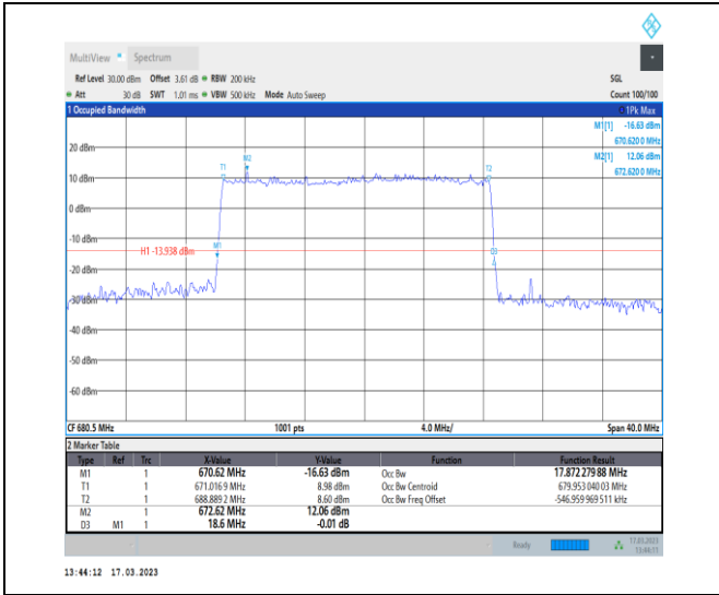
1-N71-PC3-15-20-M-4-DFT-64QAM-Outer_Full-100 @0-Ant7-17.872-18.600-≤20-PASS
