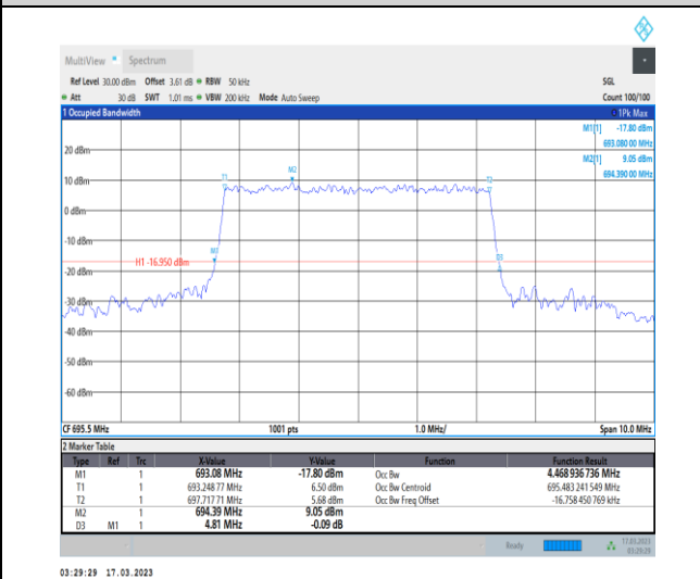
1-N71-PC3-15-5-H-6-CP-QPSK-Outer_Full-25@0-Ant7-4.469-4.810-≤5-PASS
