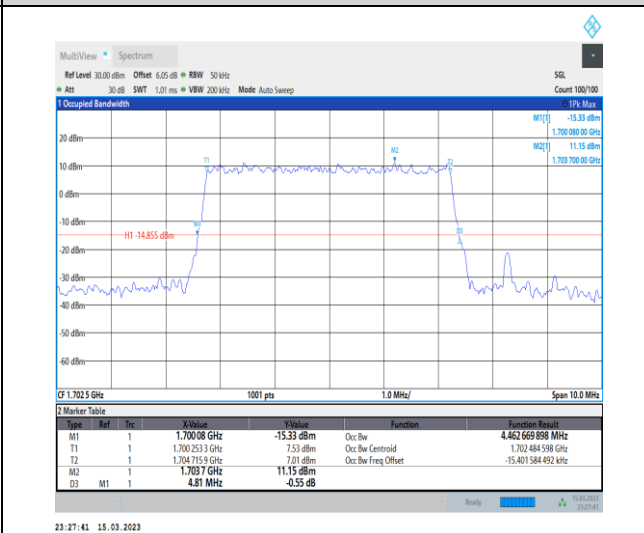
1-N70-PC3-15-5-M-3-DFT-16QAM-Outer_Full-25@0-Ant7-4.463-4.810-≤5-PASS
