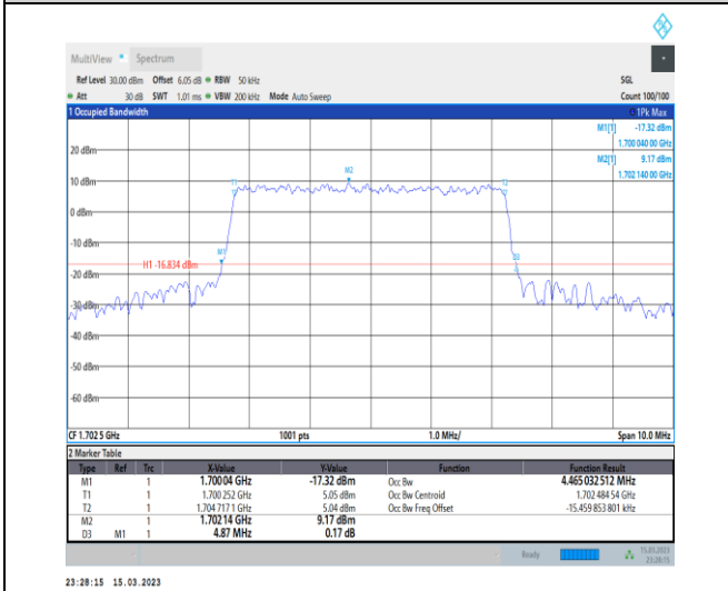
1-N70-PC3-15-5-M-6-CP-QPSK-Outer_Full-25@0-Ant7-4.465-4.870-≤5-PASS
