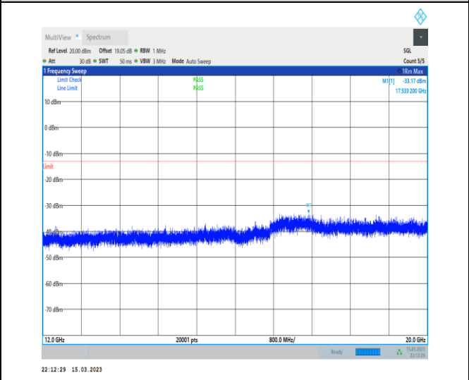
1-N66-PC3-15-40-M-1-DFT-PI2BPSK-Inner_1RB_L eft-1@1-12000-20000-Ant1-17533.20--33.17--13-PASS
