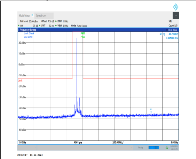
1-N66-PC3-15-40-M-1-DFT-PI2BPSK-Inner_1RB_L eft-1@1-1000-3000-Ant1-2657.00--44.79--13-PASS
