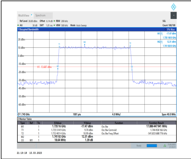
1-N66-PC3-15-20-M-3-DFT-16QAM-Outer_Full-100 @0-Ant1-17.886-18.640-≤20-PASS
