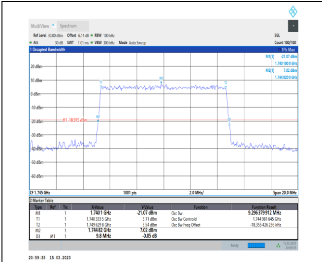
1-N66-PC3-15-10-M-9-CP-256QAM-Outer_Full-52@ 0-Ant1-9.296-9.800-≤10-PASS
