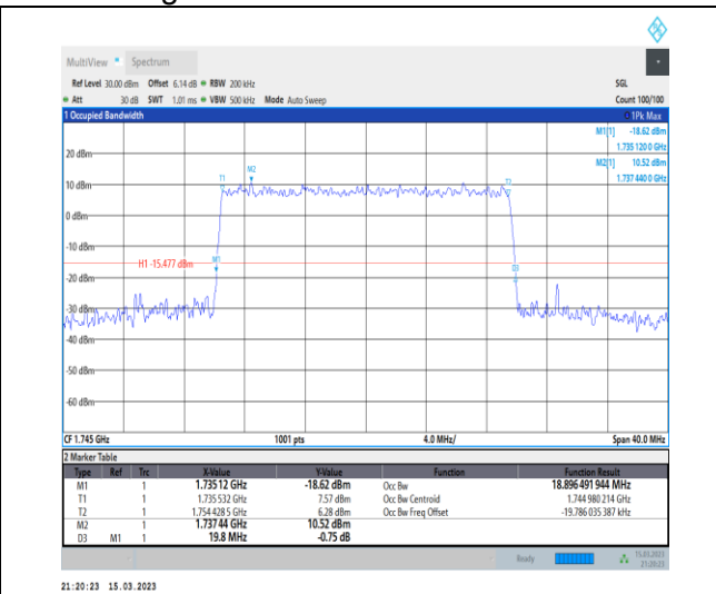
1-N66-PC3-15-20-M-8-CP-64QAM-Outer_Full-106@ 0-Ant1-18.896-19.800-≤20-PASS
