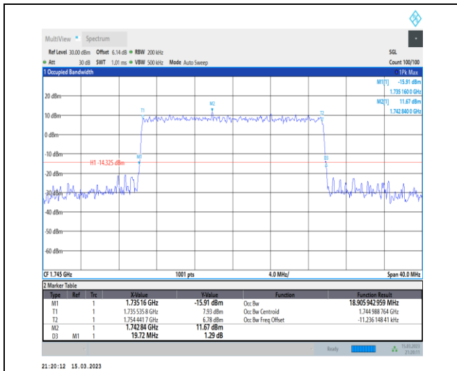
1-N66-PC3-15-20-M-7-CP-16QAM-Outer_Full-106@ 0-Ant1-18.906-19.720-≤20-PASS
