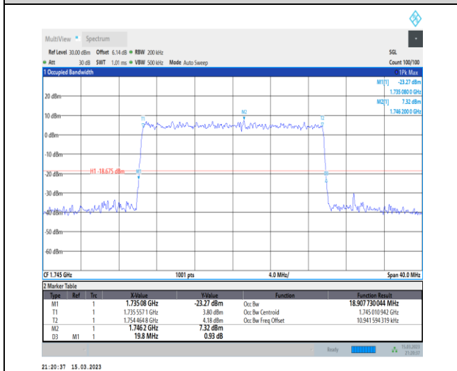
1-N66-PC3-15-20-M-9-CP-256QAM-Outer_Full-106 @0-Ant1-18.908-19.800-≤20-PASS
