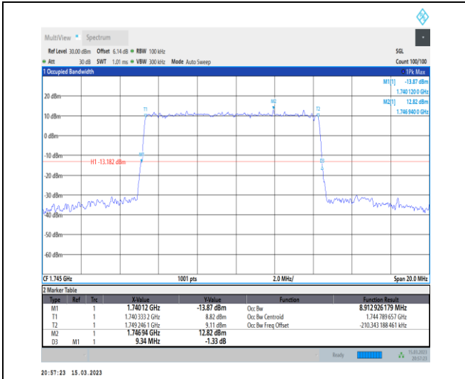
1-N66-PC3-15-10-M-1-DFT-QPSK-Outer_Full-50@0-Ant1-8.913-9.340-≤10-PASS
