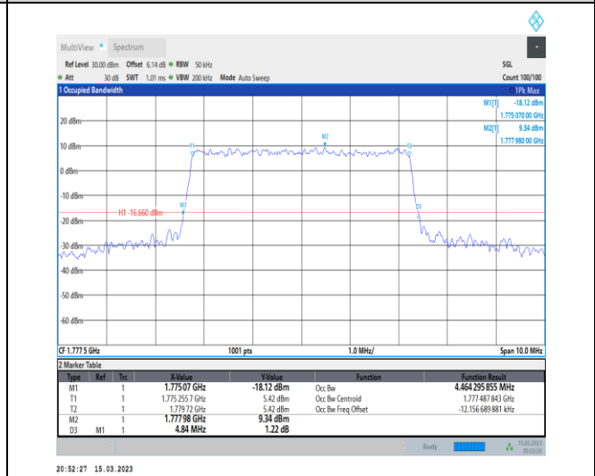
1-N66-PC3-15-5-H-6-CP-QPSK-Outer_Full-25@0-A nt1-4.464-4.840-≤5-PASS
