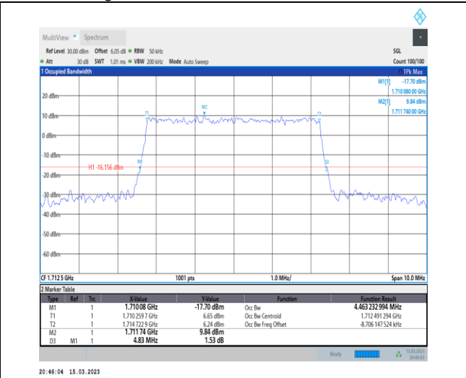
1-N66-PC3-15-5-L-6-CP-QPSK-Outer_Full-25@0-An t1-4.463-4.830-≤5-PASS
