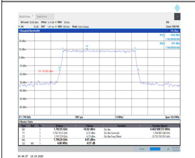
1-N66-PC3-15-5-M-6-CP-QPSK-Outer_Full-25@0-A nt1-4.464-4.860-≤5-PASS
