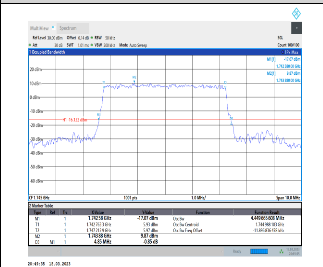
1-N66-PC3-15-5-M-7-CP-16QAM-Outer_Full-25@0- Ant1-4.45-4.850-≤5-PASS
