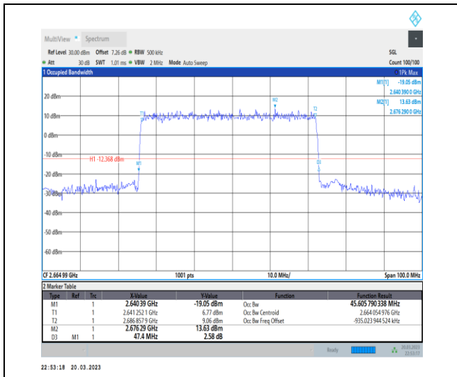
1-N41-30-50-H-4-DFT-64QAM-Outer_Full-128@0-A nt1-45.606-47.400-≤50-PASS
