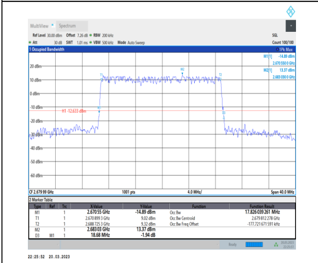
1-N41-30-20-H-3-DFT-16QAM-Outer_Full-50@0-Ant1 1-17.826-18.680-≤20-PASS
