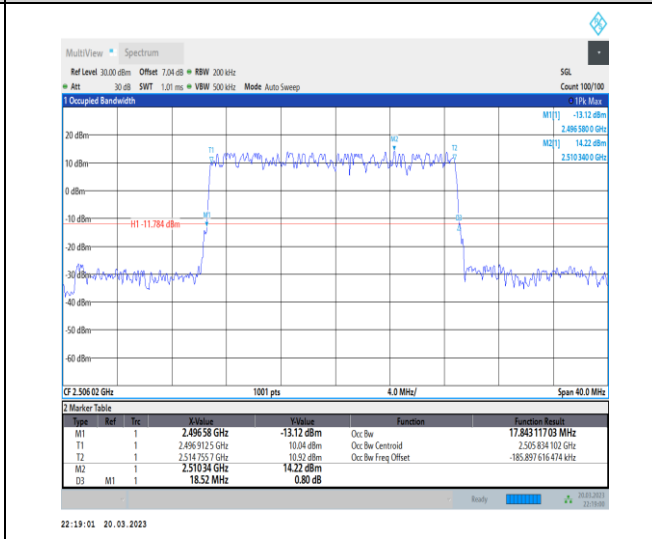
1-N41-30-20-L-2-DFT-PI2BPSK-Outer_Full-50@0-Ant1 -17.843-18.520-≤20-PASS
