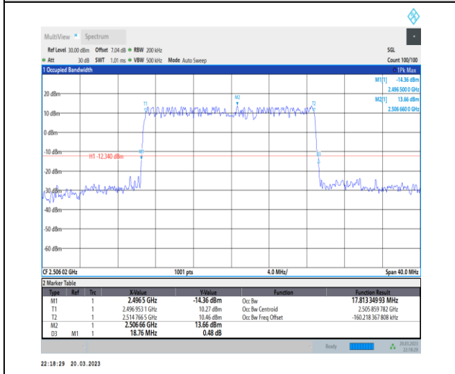
1-N41-30-20-L-1-DFT-QPSK-Outer_Full-50@0-Ant1 -17.813-18.760-≤20-PASS
