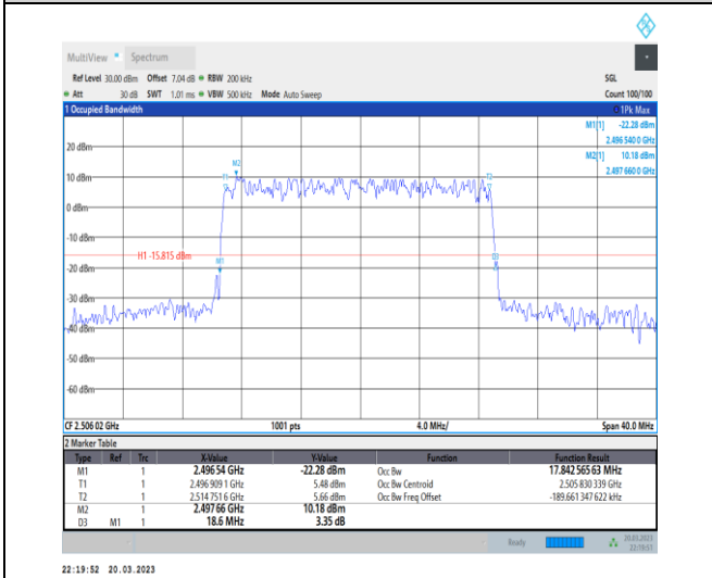
1-N41-30-20-L-5-DFT-256QAM-Outer_Full-50@0-A nt1-17.843-18.600-≤20-PASS
