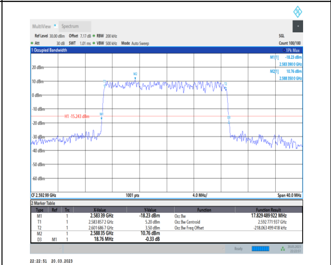
1-N41-30-20-M-5-DFT-256QAM-Outer_Full-50@0-A nt1-17.829-18.760-≤20-PASS
