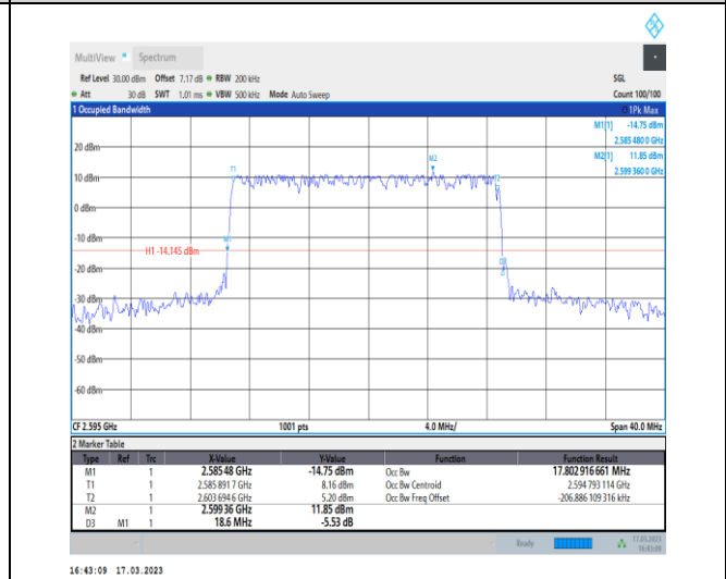
1-N38-30-20-M-5-DFT-256QAM-Outer_Full-50@0-A nt1-17.803-18.600-≤20-PASS
