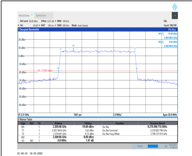
1-N30-PC3-15-10-M-9-CP-256QAM-Outer_Full-52@ 0-Ant1-9.276-9.800-≤10-PASS
