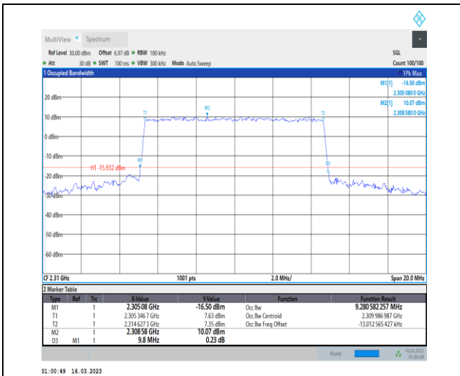
1-N30-PC3-15-10-L-6-CP-QPSK-Outer_Full-52@0-A nt1-9.281-9.800-≤10-PASS
