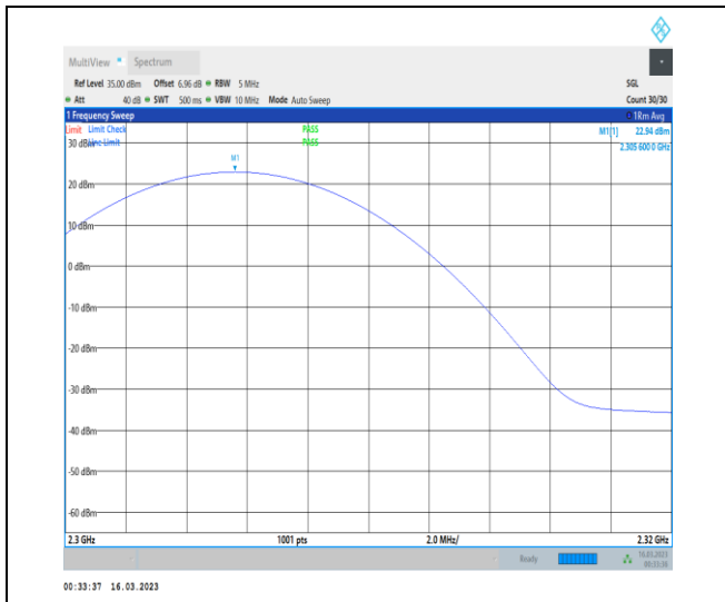
1-N30-PC3-15-10-M-1-DFT-PI2BPSK-Inner_1RB_L eft-1@1-2300-2320-Ant1-2305.60-22.94-99-PASS
