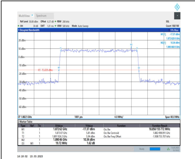
1-N25-PC3-15-20-M-7-CP-16QAM-Outer_Full-106@ 0-Ant1-18.856-19.720-≤20-PASS
