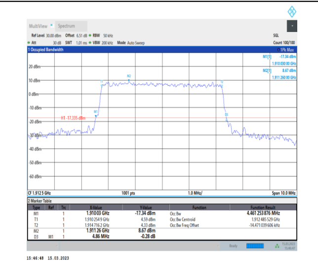
1-N25-PC3-15-5-H-6-CP-QPSK-Outer_Full-25@0-A nt1-4.461-4.860-≤5-PASS
