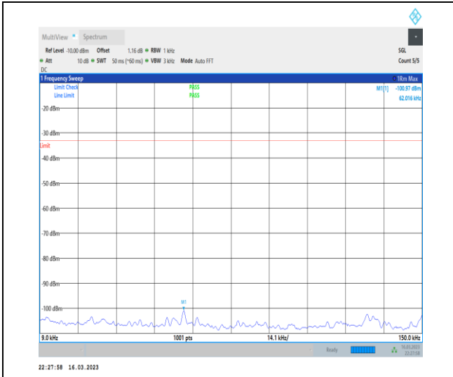
1-N14-PC3-15-10-M-1-DFT-PI2BPSK-Inner_1RB_L eft-1@1-0.009-0.15-Ant7-0.06--100.97--33-PASS
