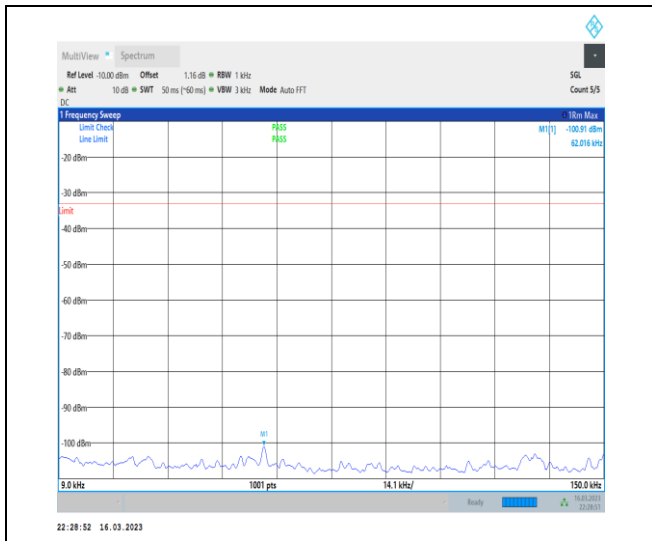
1-N14-PC3-15-10-H-1-DFT-PI2BPSK-Inner_1RB_L eft-1@1-0.009-0.15-Ant7-0.06--100.91--33-PASS
