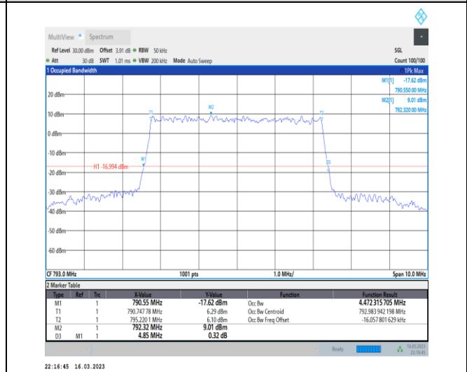
1-N14-PC3-15-5-M-7-CP-16QAM-Outer_Full-25@0-Ant7-4.472-4.850-≤5-PASS
