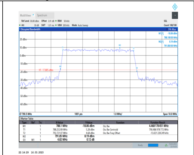
1-N14-PC3-15-5-L-6-CP-QPSK-Outer_Full-25@0-An t7-4.468-4.820-≤5-PASS
