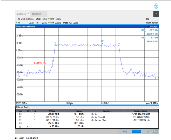
1-N14-PC3-15-5-M-6-CP-QPSK-Outer_Full-25@0-Ant7-4.466-4.810-≤5-PASS
