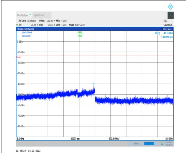
1-N12-PC3-15-15-M-1-DFT-PI2BPSK-Inner_1RB_L eft-1@1-3000-12000-Ant7-7431.15--43.18--13-PAS S
