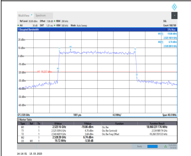
1-N7-PC3-15-20-M-9-CP-256QAM-Outer_Full-106@0 0-Ant1-18.96-19.720-≤20-PASS
