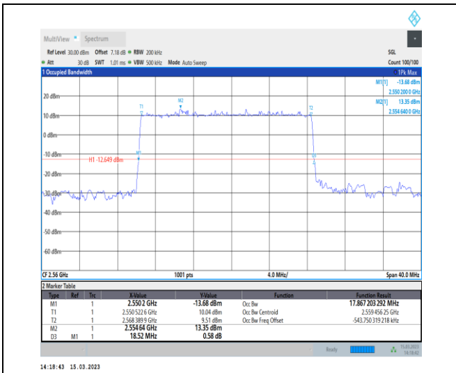
1-N7-PC3-15-20-H-2-DFT-PI2BPSK-Outer_Full-100 @0-Ant1-17.867-18.520-≤20-PASS
