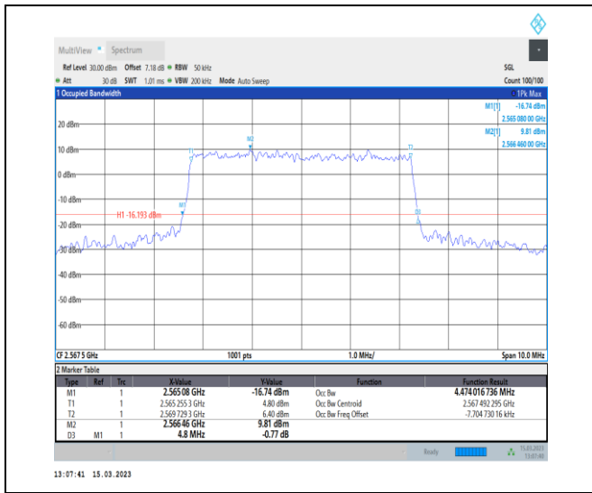
1-N7-PC3-15-5-H-7-CP-16QAM-Outer_Full-25@0-A nt1-4.474-4.800-≤5-PASS
