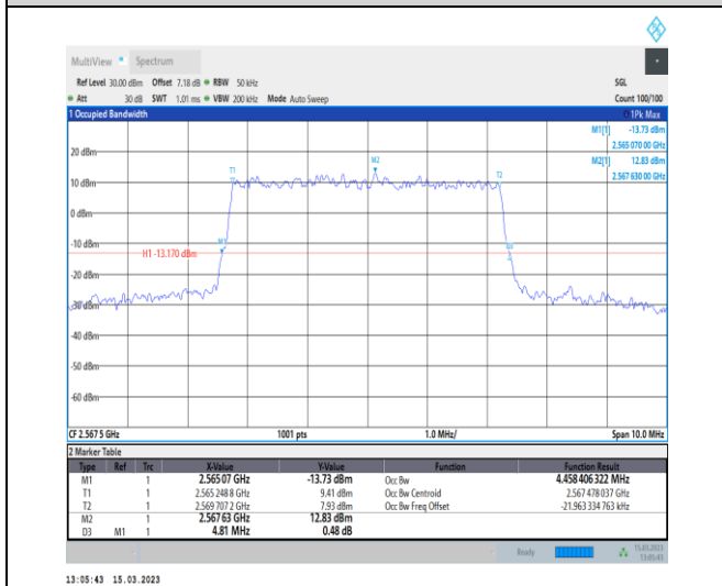
1-N7-PC3-15-5-H-1-DFT-QPSK-Outer_Full-25@0-A nt1-4.458-4.810-≤5-PASS
