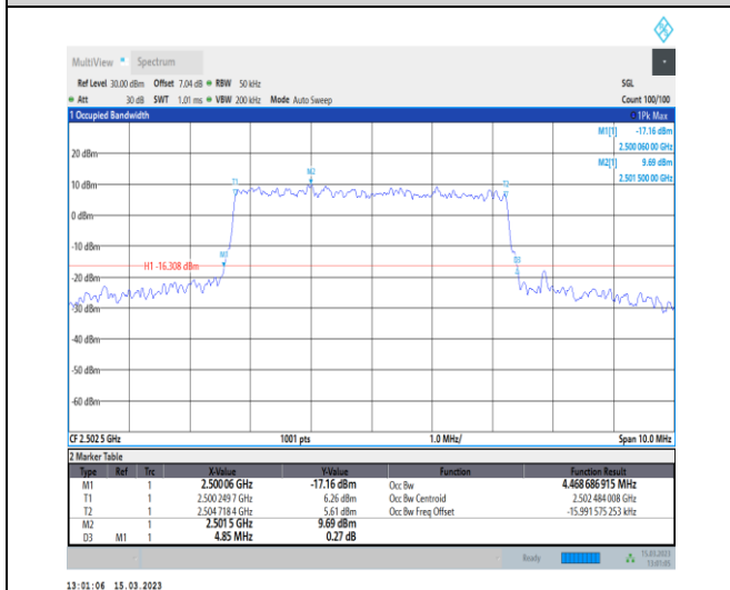
1-N7-PC3-15-5-L-7-CP-16QAM-Outer_Full-25@0-Ant1-4.469-4.850-≤5-PASS
