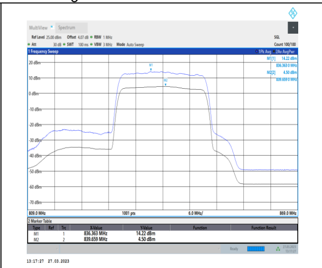
1-N5-PC3-15-20-H-2-CP-256QAM-Outer_Full-106@ 0-Ant1-9.72-100%-0.00-9.72-PASS-≤13
