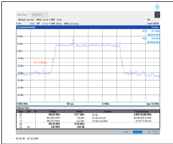
1-N5-PC3-15-5-H-7-CP-16QAM-Outer_Full-25@0-A nt1-4.469-4.830-≤5-PASS
