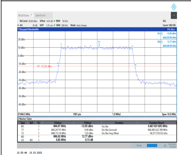
1-N5-PC3-15-5-H-1-DFT-QPSK-Outer_Full-25@0-A nt1-4.467-4.830-≤5-PASS
