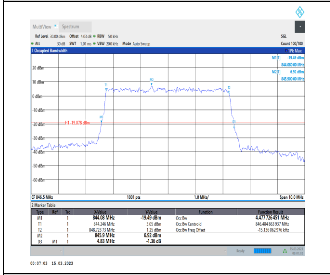
1-N5-PC3-15-5-H-9-CP-256QAM-Outer_Full-25@0-A Ant1-4.478-4.830-≤5-PASS
