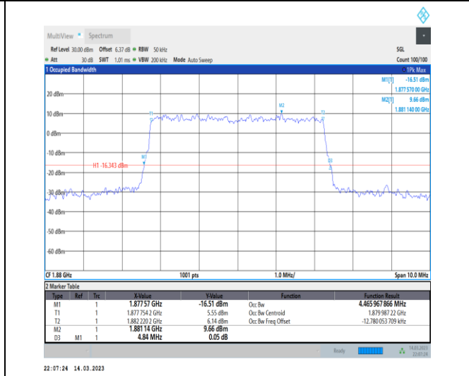
1-N2-PC3-15-5-M-7-CP-16QAM-Outer_Full-25@0-A nt1-4.466-4.840-≤5-PASS
