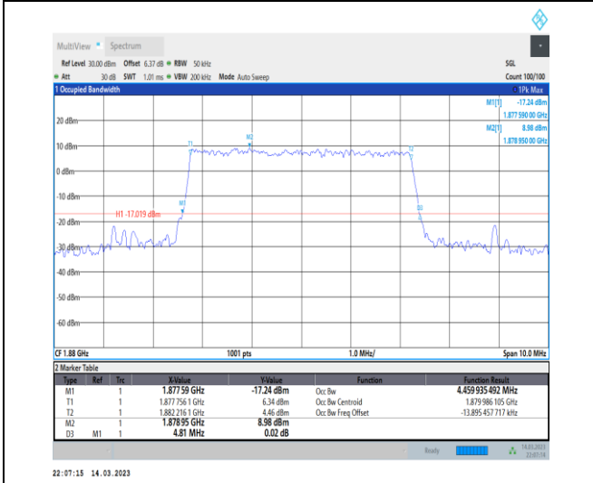
1-N2-PC3-15-5-M-6-CP-QPSK-Outer_Full-25@0-An t1-4.46-4.810-≤5-PASS
