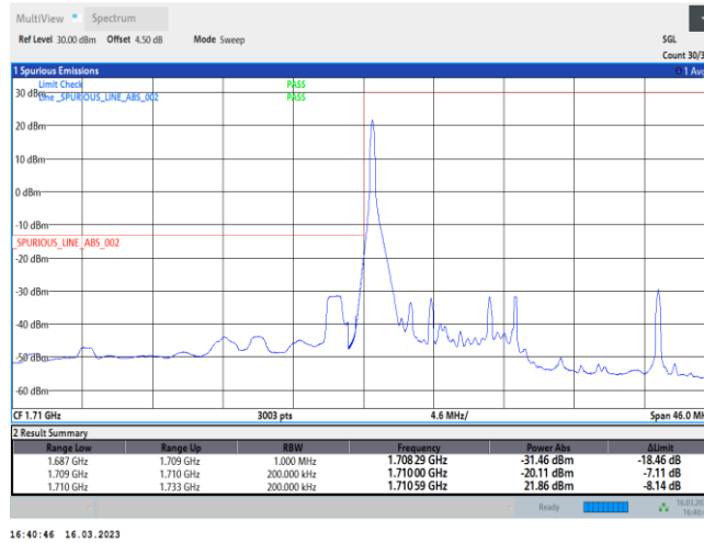
66-66-10MHz-10MHz-QPSK-QPSK-132022-132121-50RB#0-50RB#0
