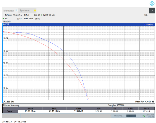
38-38-20MHz-20MHz-QPSK-QPSK-37901-38099-100RB#0-100RB#0
