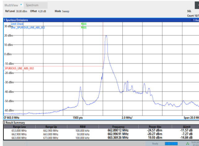
Band71-5MHz-QPSK-133147-25RB#0
