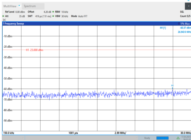
Band71-20MHz-QPSK-133222-1RB#0-Range2:0.15~30MHz
