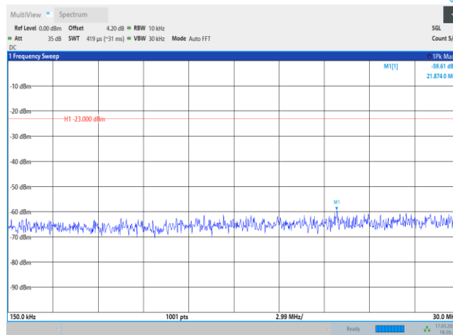
Band14-10MHz-QPSK-23330-1RB#0-Range2:0.15~30MHz
