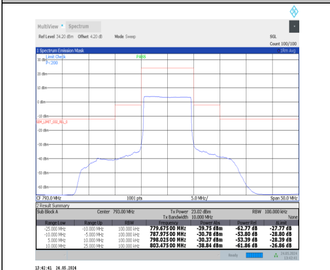
NTNV-Band14-10MHz-QPSK-23330-50RB#0--25.00--10.0 0-PASS
