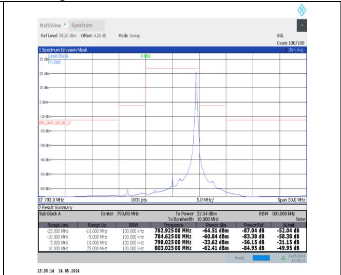
NTNV-Band14-10MHz-QPSK-23330-1RB#49--25.00--10.0 0-PASS
