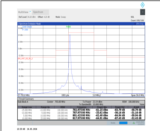
NTNV-Band14-10MHz-QPSK-23330-1RB#0--25.00--10.0 -PASS
