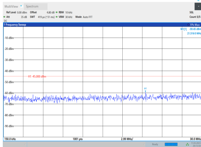
Band7-20MHz-QPSK-20850-1RB#0-Range2:0.15~30MHz
