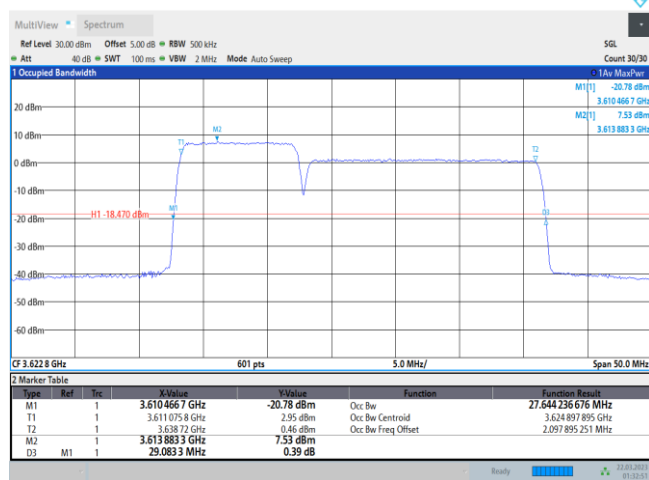
48-48-10MHz-20MHz-QPSK-QPSK-55896-56040-50RB#0-100RB#0
