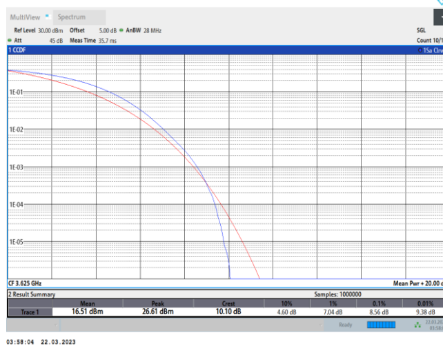
48-48-20MHz-20MHz-QPSK-QPSK-55891-56089-100RB#0-100RB#0
