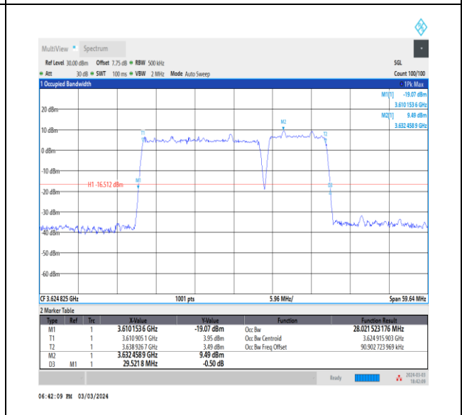
NTVN_CA_n48B_PC3_30+30_20+10_M+M_Ant0_TID2_1_#1
