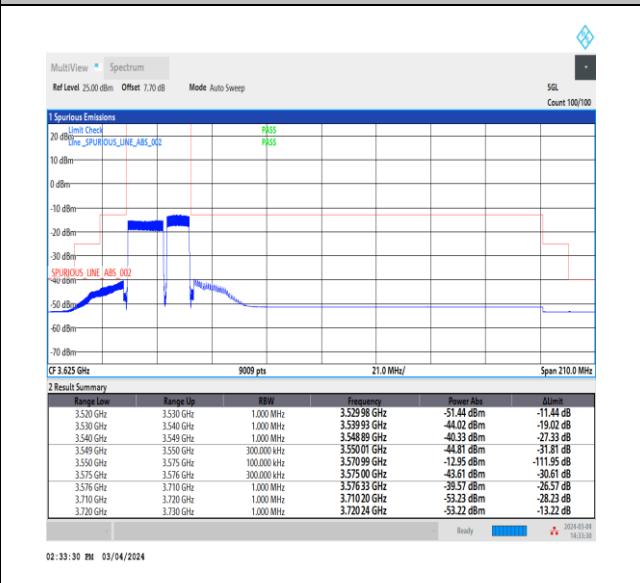
NTNV_CA_n48B_PC3_30+30_15+10_L+L_TID6_1_#1
