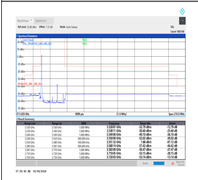
NTNV_CA_n48B_PC3_30+30_20+10_L+L_TID4_1_#1
