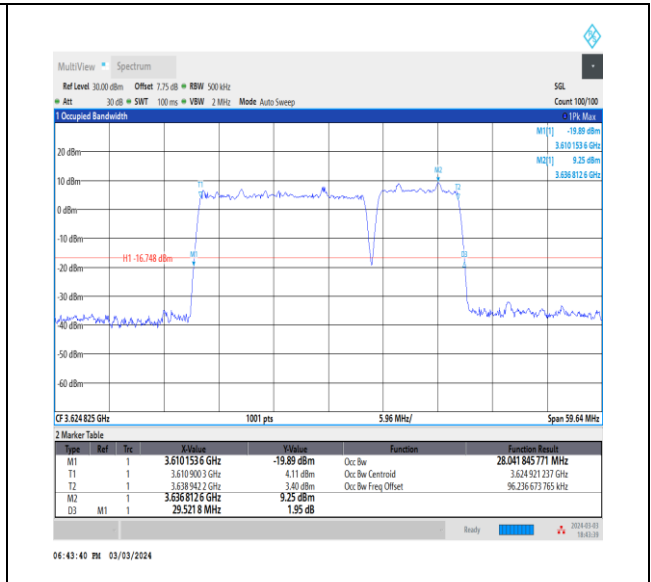
NTNV_CA_n48B_PC3_30+30_20+10_M+M_Ant0_TID8_1_#1
