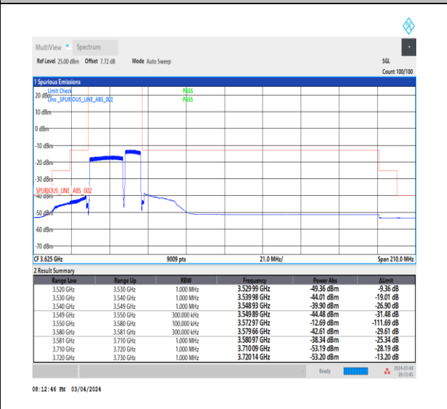
NTNV_CA_n48B_PC3_30+30_20+10_L+L_TID6_1_#1
