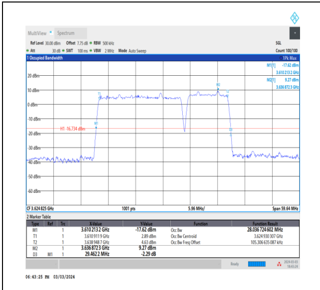
NTNV_CA_n48B_PC3_30+30_20+10_M+M_Ant0_TID7_1_#1
