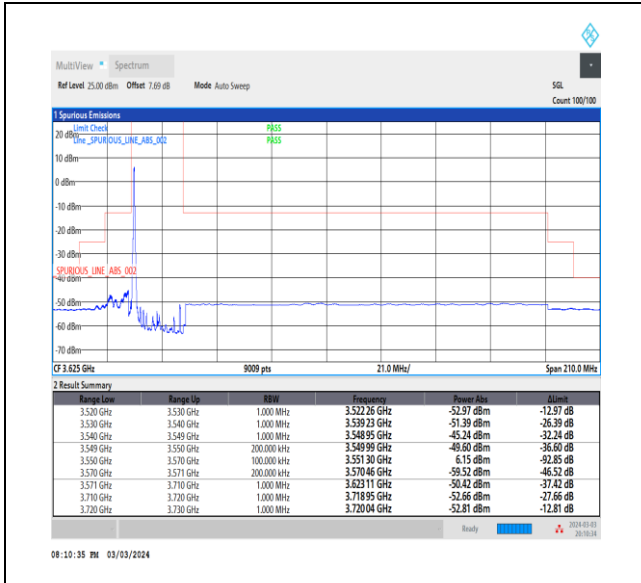
NTNV_CA_n48B_PC3_30+30_10+10_L+L_TID1_1_#1
