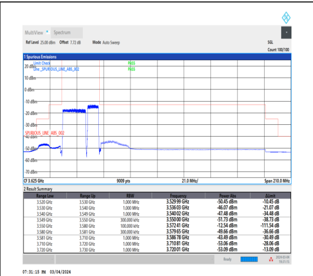
NTNV_CA_n48B_PC3_30+30_20+10_L+L_TID3_1_#1
