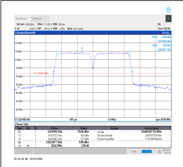
NTNV_CA_n48B_PC3_30+30_10+10_M+M_Ant0_TID5_1_#1
