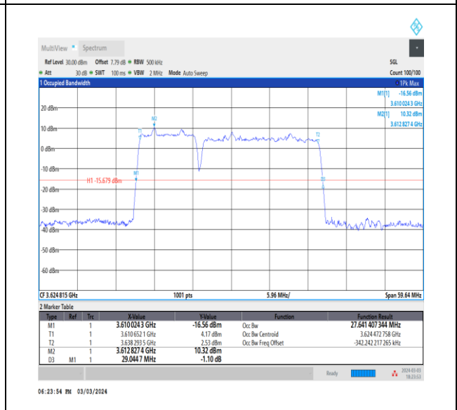
NTVN_CA_n48B_PC3_30+30_10+20_M+M_Ant0_TID2_1_#1
