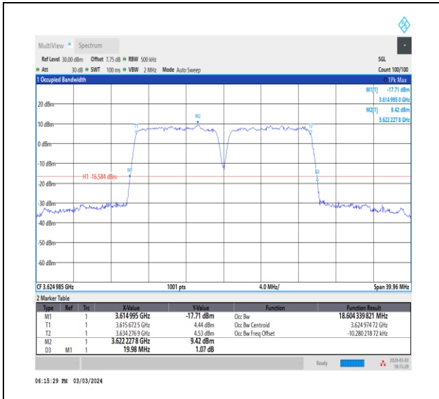
NTNV_CA_n48B_PC3_30+30_10+10_M+M_Ant0_TID9_1_#1
