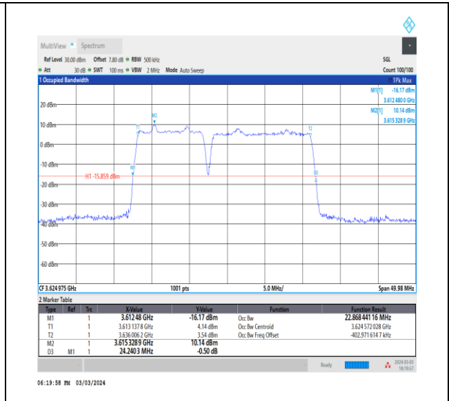
NTVN_CA_n48B_PC3_30+30_10+15_M+M_Ant0_TID9_1_#1
