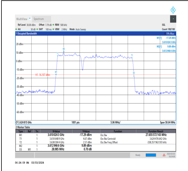
NTNV_CA_n48B_PC3_30+30_10+20_M+M_Ant0_TID3_1_#1
