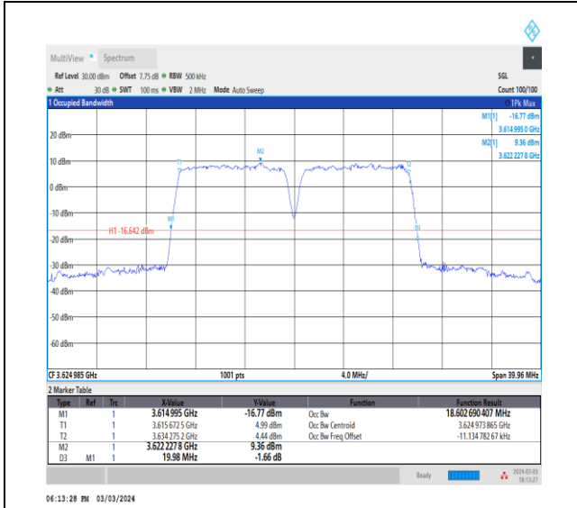
NTNV_CA_n48B_PC3_30+30_10+10_M+M_Ant0_TID1_1_#1
