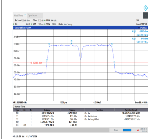
NTNV_CA_n48B_PC3_30+30_10+10_M+M_Ant0_TID3_1_#1
