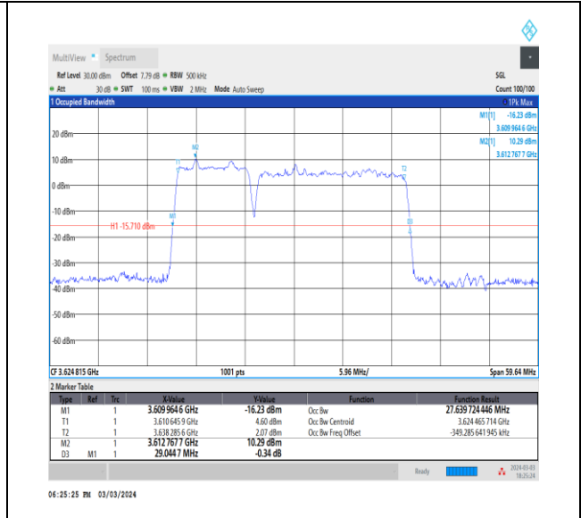
NTNV_CA_n48B_PC3_30+30_10+20_M+M_Ant0_TID8_1_#1
