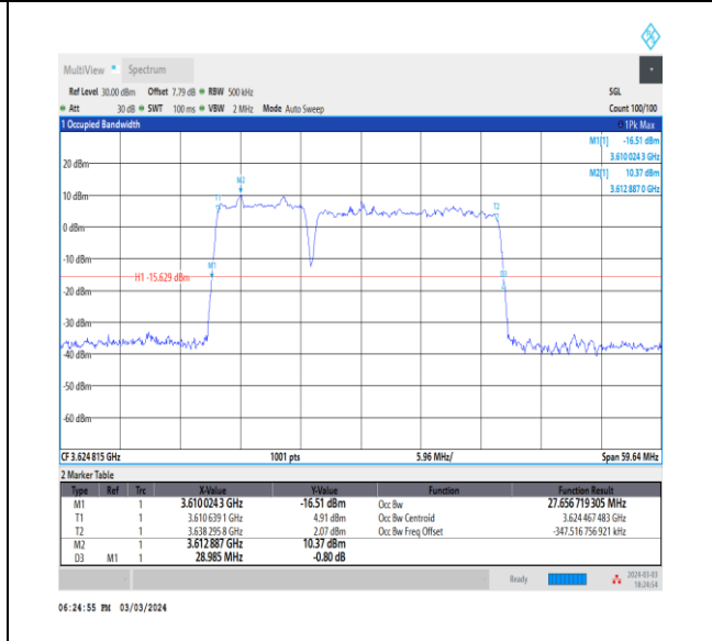
NTNV_CA_n48B_PC3_30+30_10+20_M+M_Ant0_TID6_1_#1
