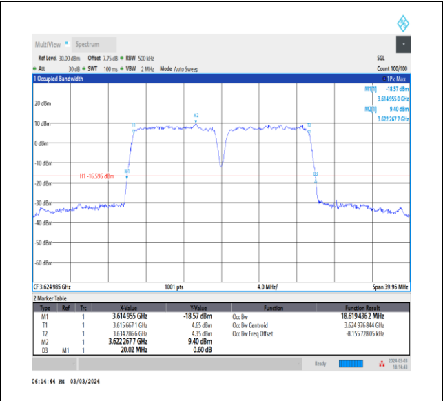
NTNV_CA_n48B_PC3_30+30_10+10_M+M_Ant0_TID6_1_#1
