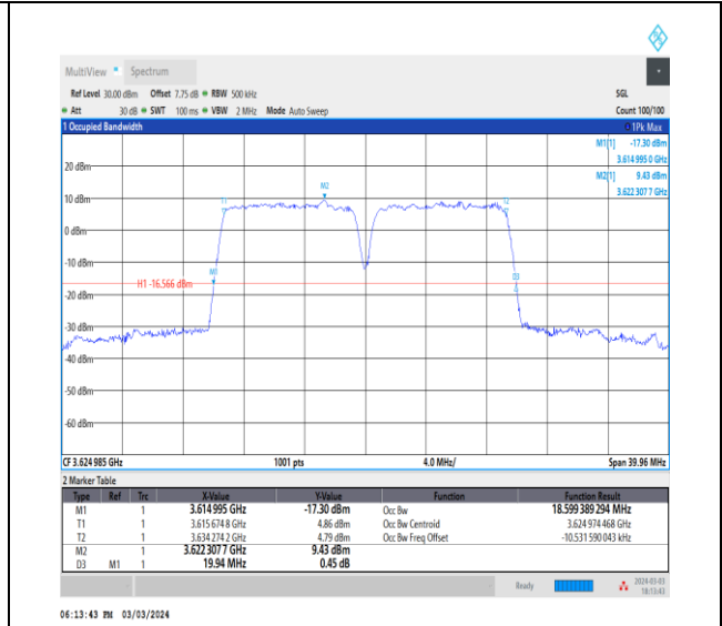
NTNV_CA_n48B_PC3_30+30_10+10_M+M_Ant0_TID2_1_#1
