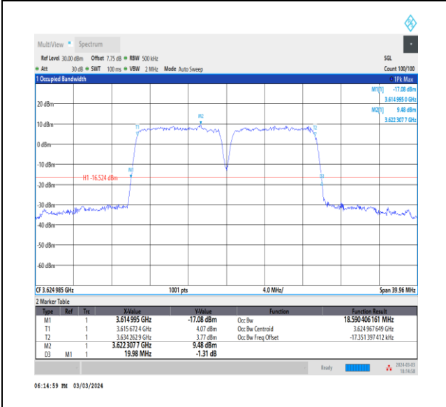
NTNV_CA_n48B_PC3_30+30_10+10_M+M_Ant0_TID7_1_#1
