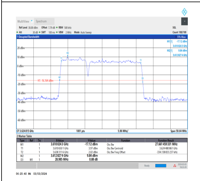
NTNV_CA_n48B_PC3_30+30_10+20_M+M_Ant0_TID9_1_#1
