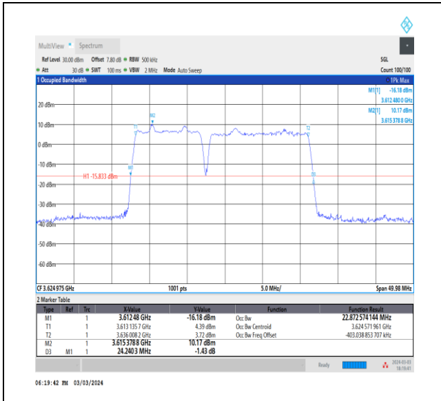
NTVN_CA_n48B_PC3_30+30_10+15_M+M_Ant0_TID8_1_#1
