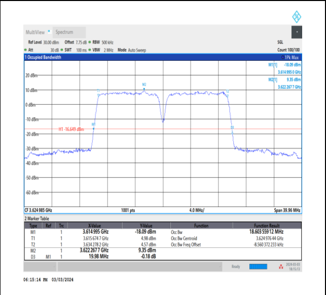
NTNV_CA_n48B_PC3_30+30_10+10_M+M_Ant0_TID8_1_#1
