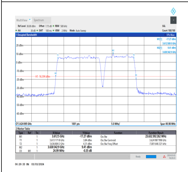
NTNV_CA_n48B_PC3_30+30_15+10_M+M_Ant0_TID8_1_#1
