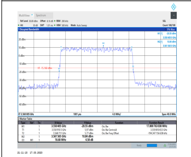
1-N48-PC3-30-20-L-3-DFT-16QAM-Outer_Full-50@0-Ant0-17.801-18.680-≤20-PASS
