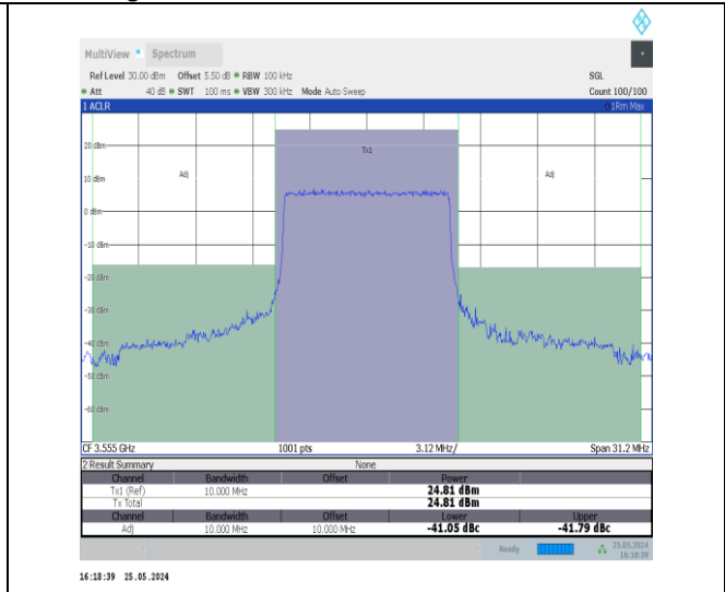
Band48-10MHz-QPSK-55290-50RB#0-PASS
