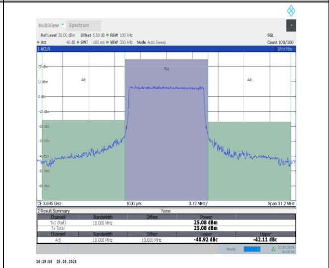
Band48-10MHz-QPSK-56690-50RB#0-PASS
