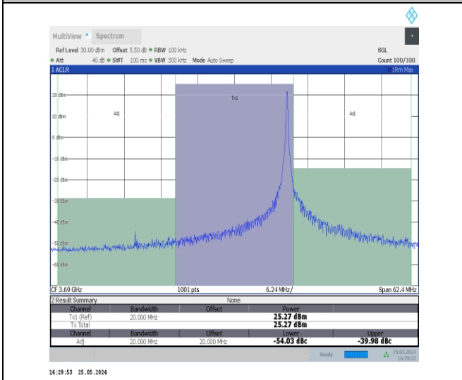
Band48-20MHz-QPSK-56640-1RB#99-PASS
