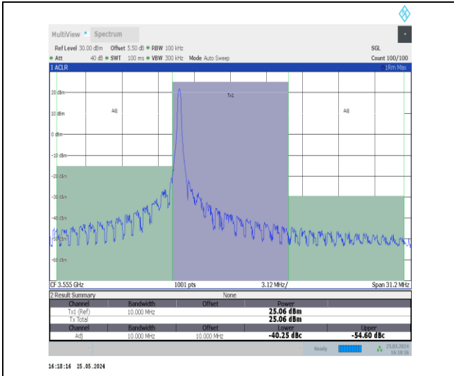
Band48-10MHz-QPSK-55290-1RB#0-PASS
