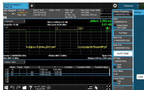
NTNV-BLE_500K-Ant1-2480
