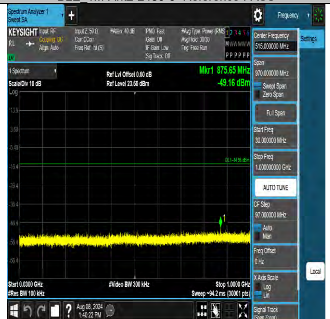
BLE 1M-Ant2-2480-30~1000-PASS
