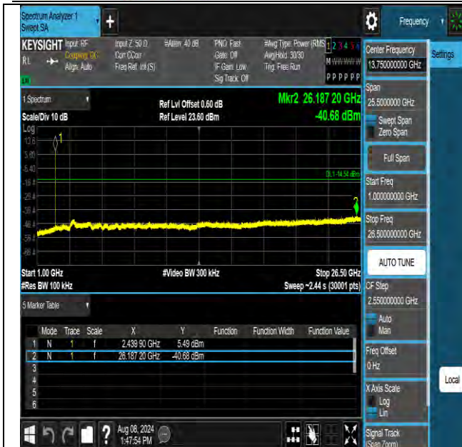
BLE 2M-Ant2-2440-1000~26500-PASS
