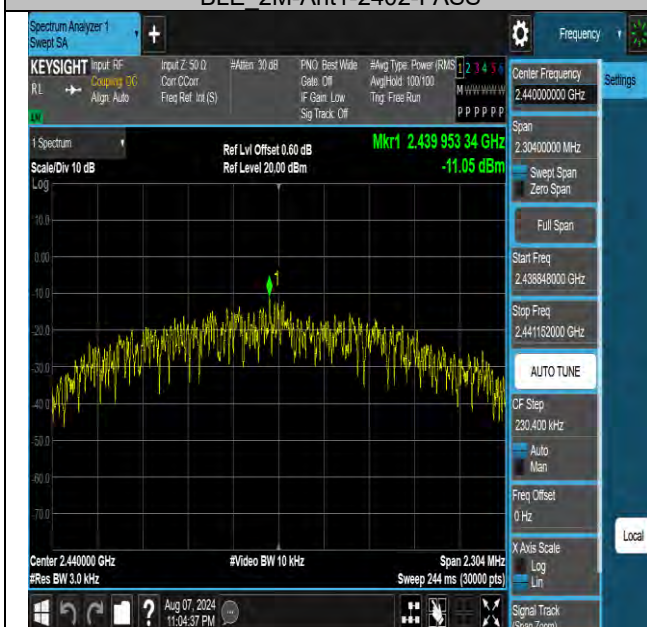
BLE 2M-Ant1-2440-PASS
