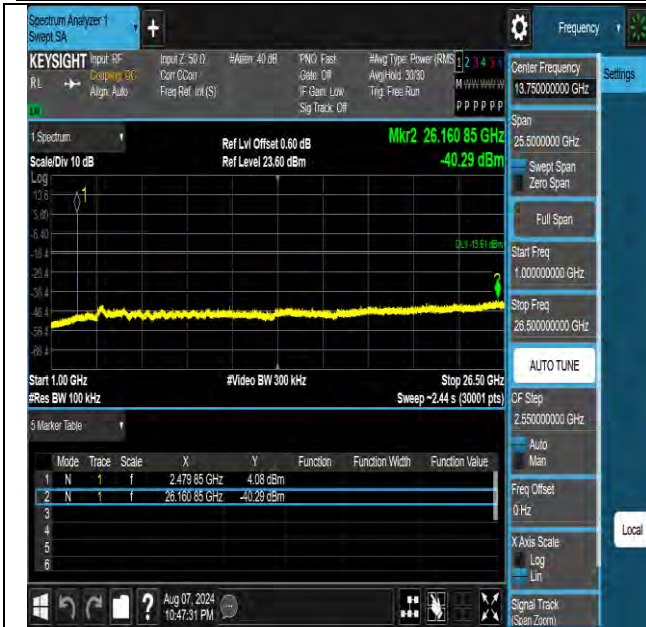
BLE 1M-Ant1-2480-1000~26500-PASS
