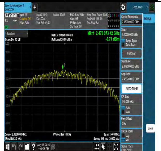
BLE 1M-Ant2-2480-PASS
