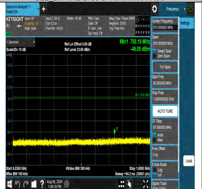
BLE 2M-Ant2-2480-30~1000-PASS
