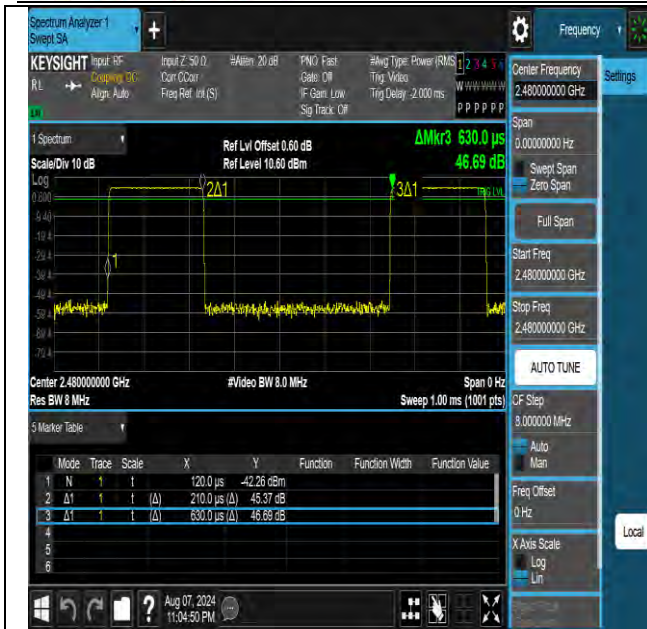
NTNV-BLE_2M-Ant1-2480
