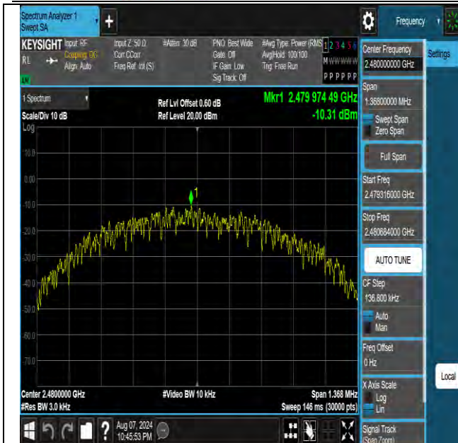
BLE 1M-Ant1-2480-PASS
