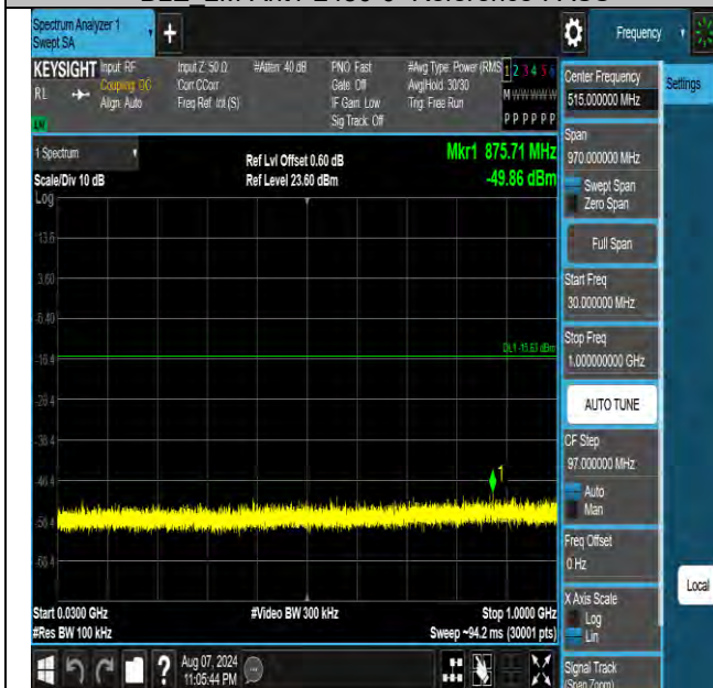
BLE 2M-Ant1-2480-30~1000-PASS
