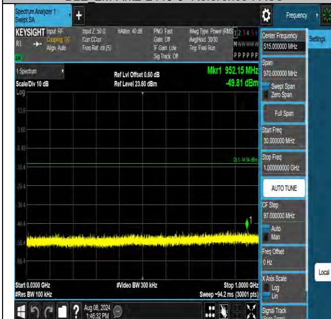
BLE 2M-Ant2-2440-30~1000-PASS
