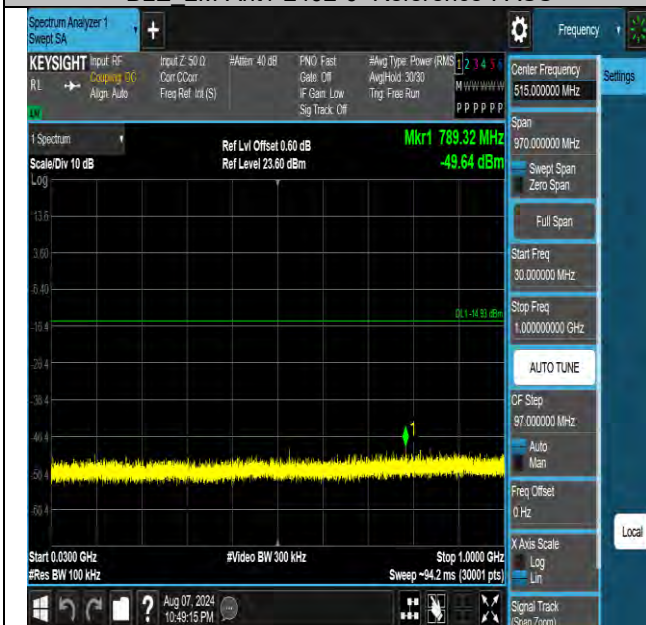
BLE 2M-Ant1-2402-30~1000-PASS
