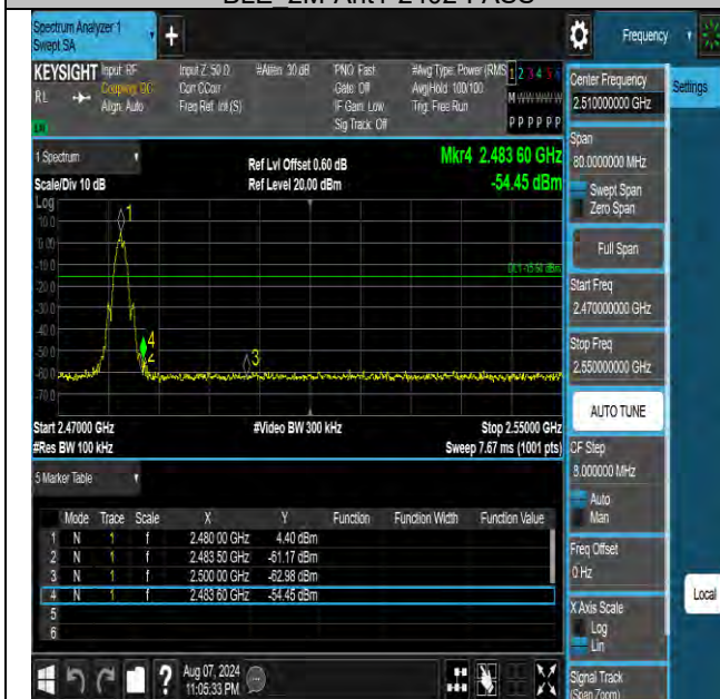
BLE 2M-Ant1-2480-PASS
