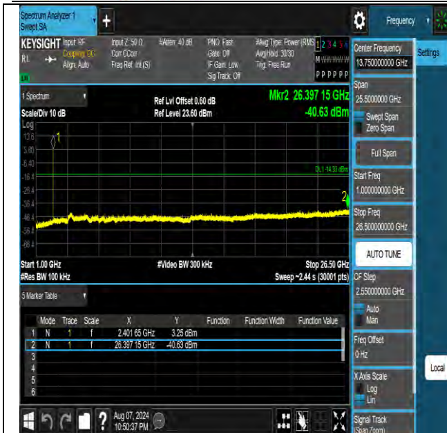
BLE 2M-Ant1-2402-1000~26500-PASS
