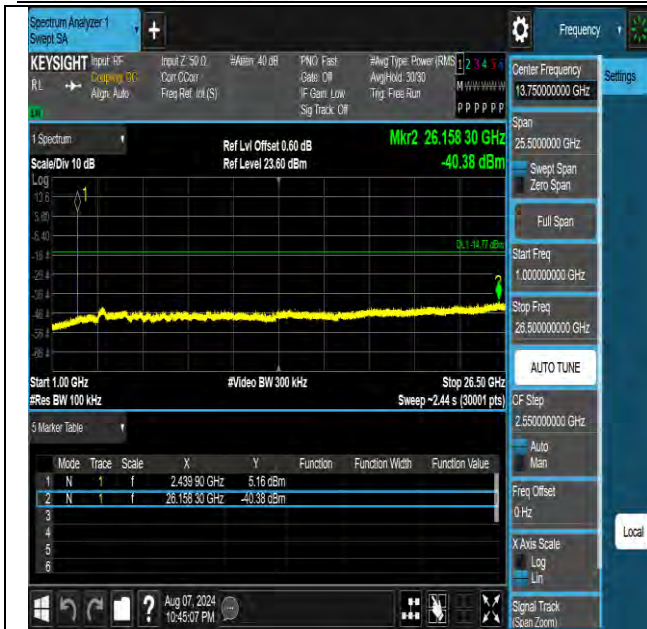
BLE 1M-Ant1-2440-1000~26500-PASS
