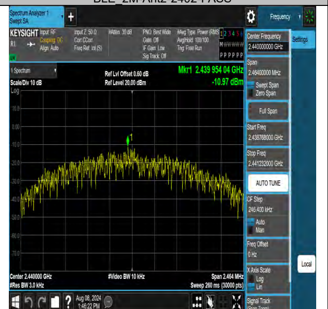
BLE 2M-Ant2-2440-PASS
