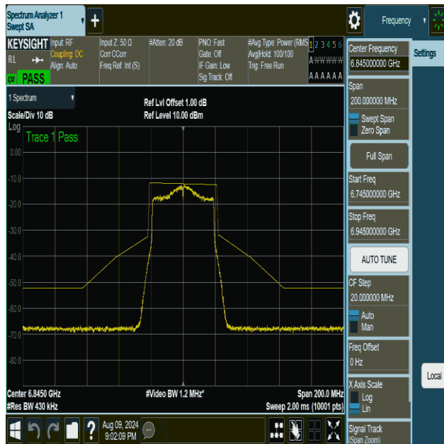
NTVN-11be40MIMO-Ant1-6845-PASS
