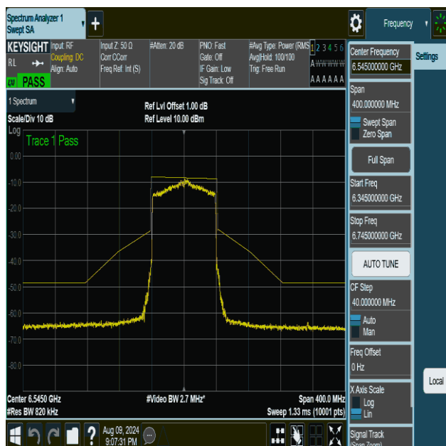
NTVN-11be80MIMO-Ant1-6545-PASS
