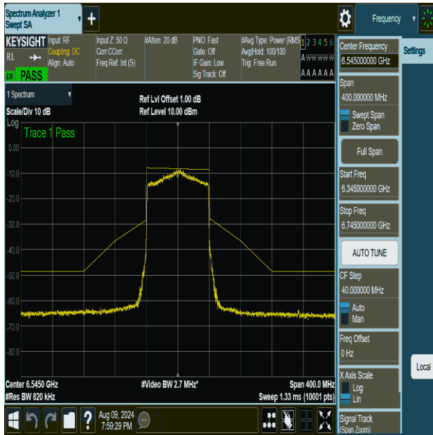
NTVN-11ax80MIMO-Ant1-6545-PASS
