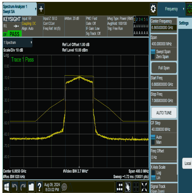
NTVN-11ax80MIMO-Ant1-6865-PASS
