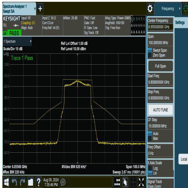
NTVN-11ax20MIMO-Ant1-6855-PASS
