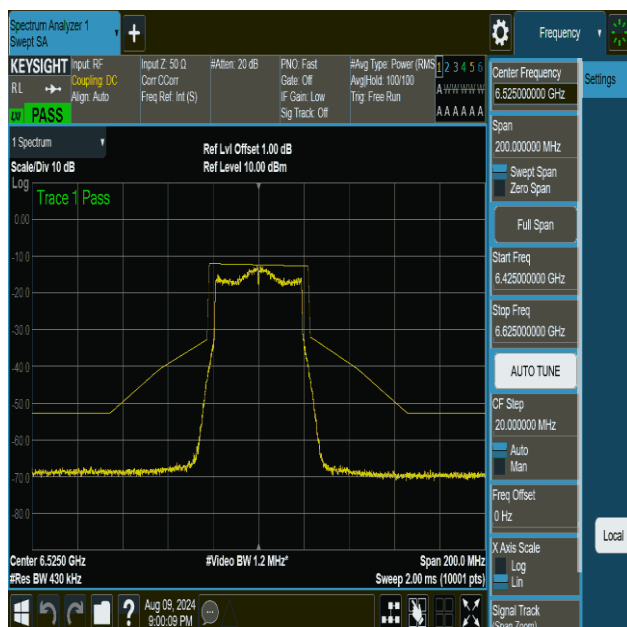
NTVN-11be40MIMO-Ant1-6525-PASS
