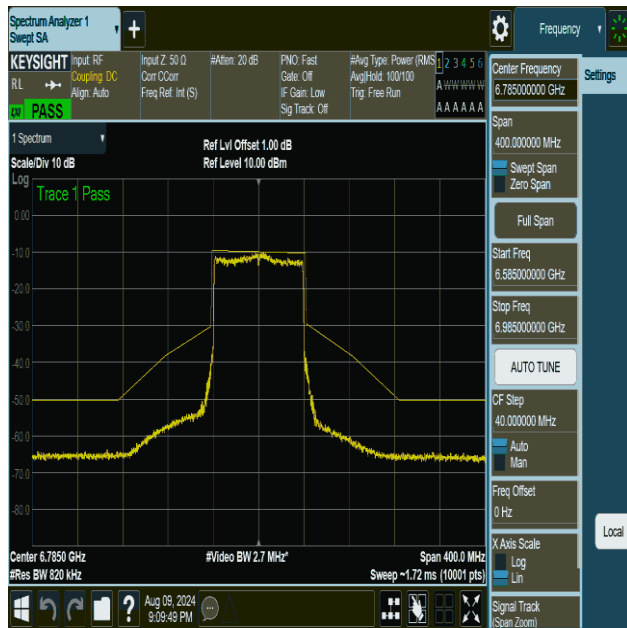
NTVN-11be80MIMO-Ant1-6785-PASS
