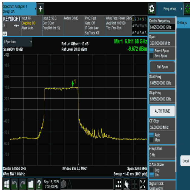
11be160MIMO-Ant1-6825-996Tone-RU67-PASS
