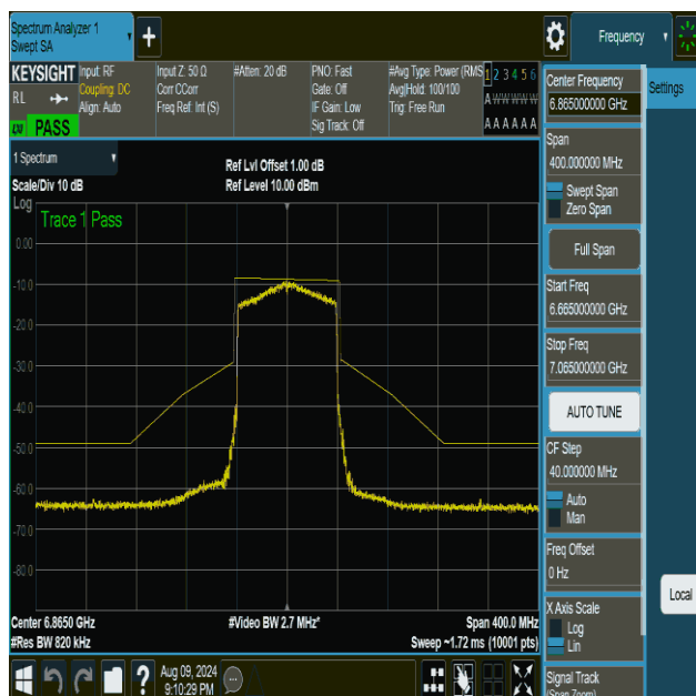
NTVN-11be80MIMO-Ant1-6865-PASS
