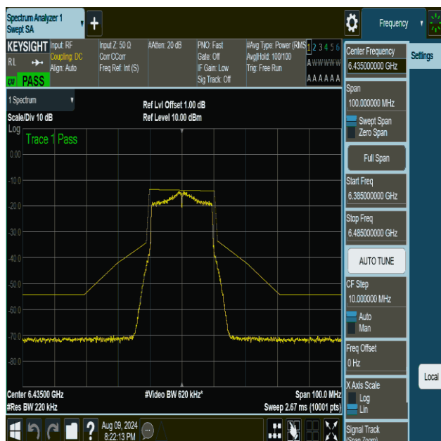
NTVN-11be20MIMO-Ant1-6435-PASS
