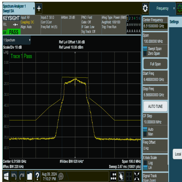
NTVN-11a-CDD-Ant1-6515-PASS
