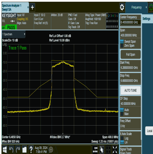
NTVN-11ax80MIMO-Ant1-6465-PASS
