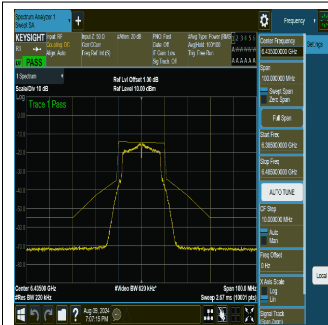
NTNV-11a-CDD-Ant1-6435-PASS
