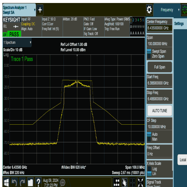
NTVN-11ax20MIMO-Ant1-6435-PASS
