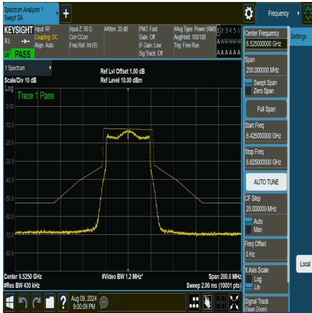
NTVN-11be40MIMO-Ant1-6525-PASS
