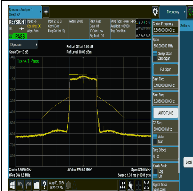
NTNV-11be160MIMO-Ant1-6505-PASS
