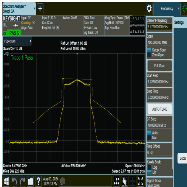
NTNV-11be20MIMO-Ant1-6475-PASS
