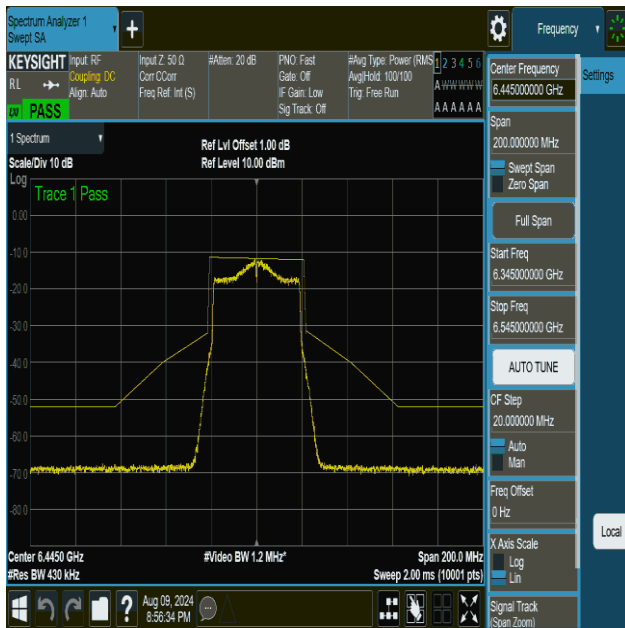
NTVN-11be40MIMO-Ant1-6445-PASS
