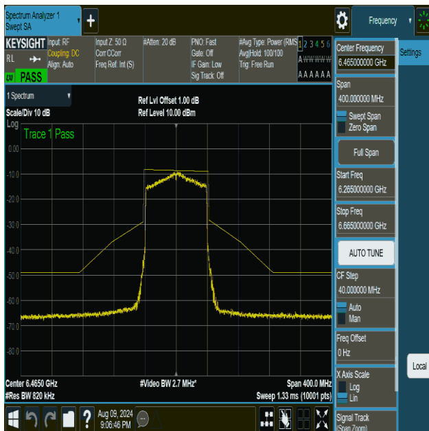
NTVN-11be80MIMO-Ant1-6465-PASS
