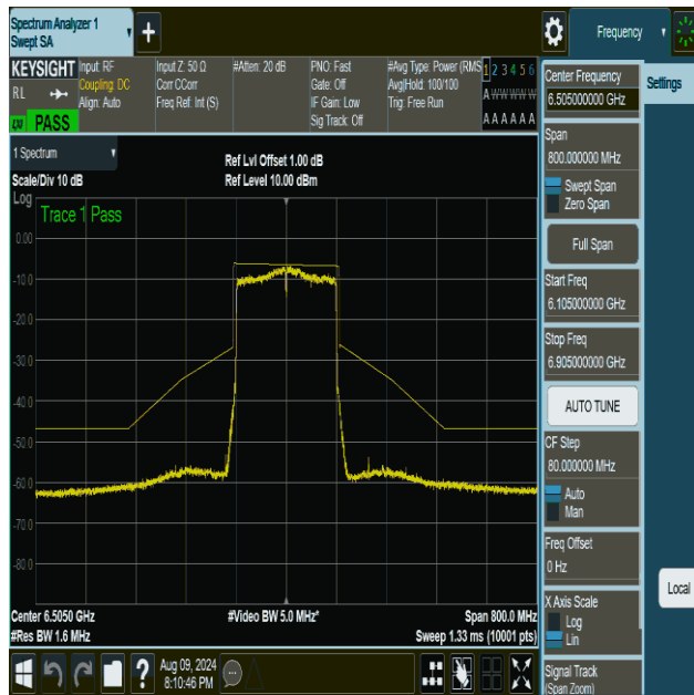
NTVN-11ax160MIMO-Ant1-6505-PASS
