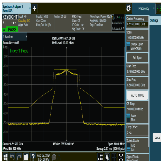
NTNV-11be20MIMO-Ant1-6515-PASS
