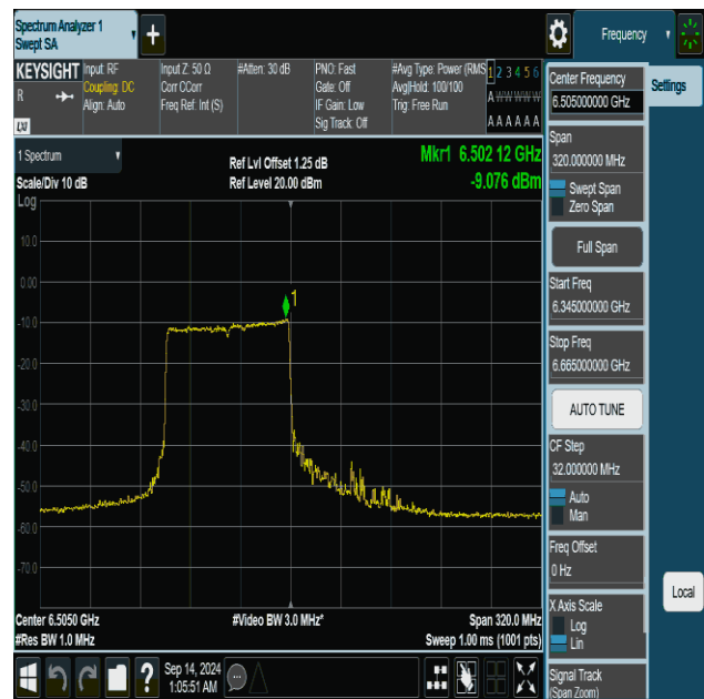
11be160MIMO-Ant1-6505-996Tone-RU67-PASS
