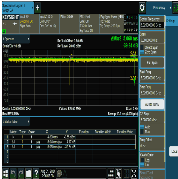
NTVN-11be160MIMO-Ant1-6025
