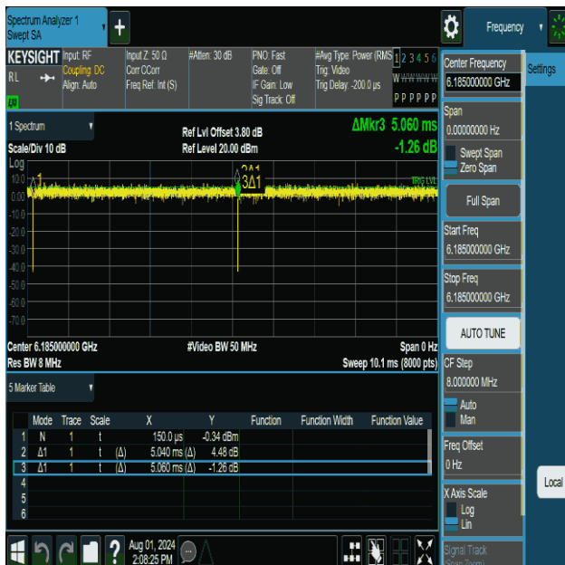
NTVN-11be160MIMO-Ant1-6185
