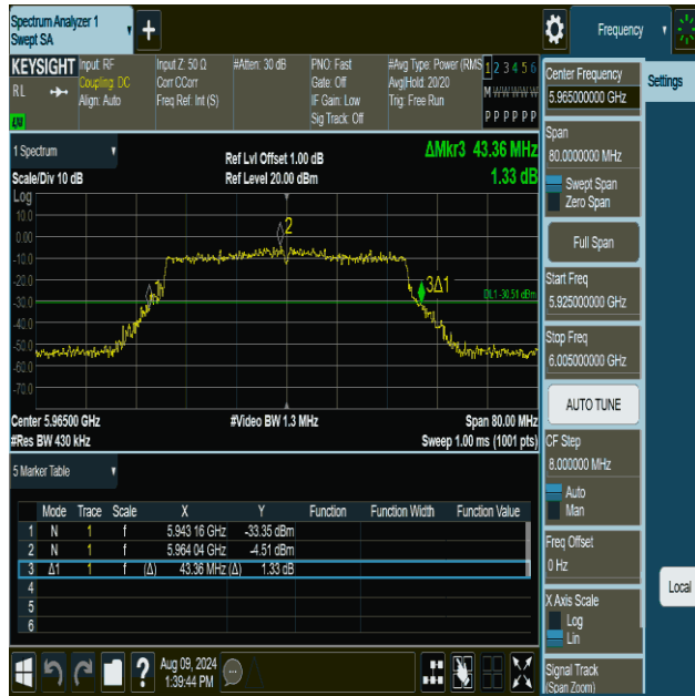
11ax40MIMO-Ant1-5965
