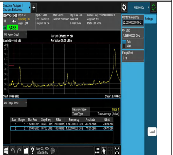
Band2_20MHz_QPSK_18700_1RB#99
