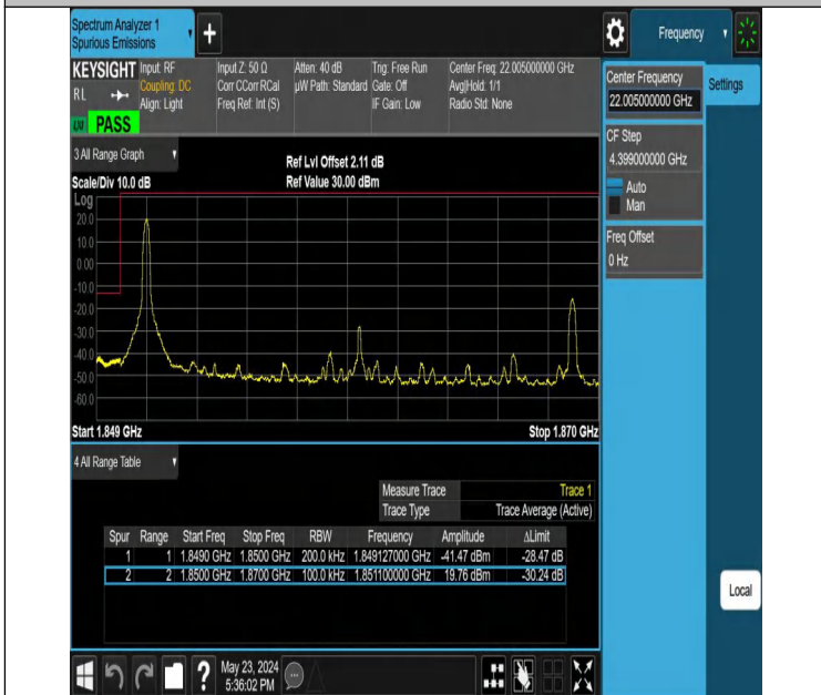
Band2_20MHz_QPSK_18700_1RB#0
