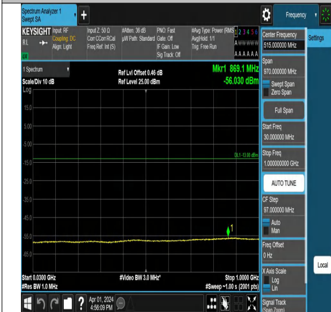
Band4-1513-3-30~1000MHz-PASS
