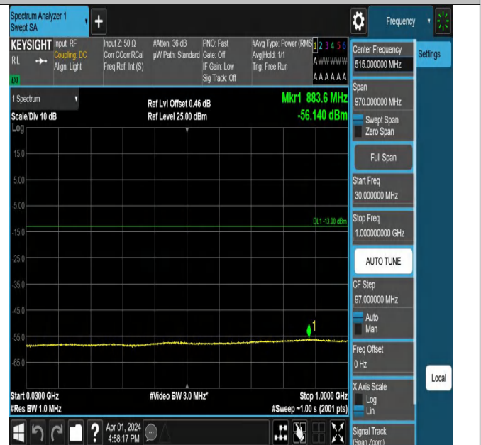
Band4-1513-4-30~1000MHz-PASS
