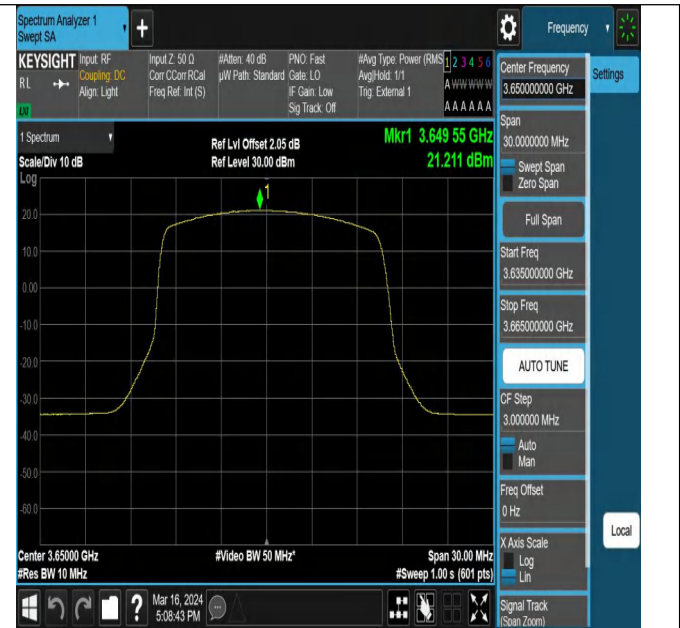
43(3600-3700)-15MHz-16QAM-44090-1RB#38-PASS
