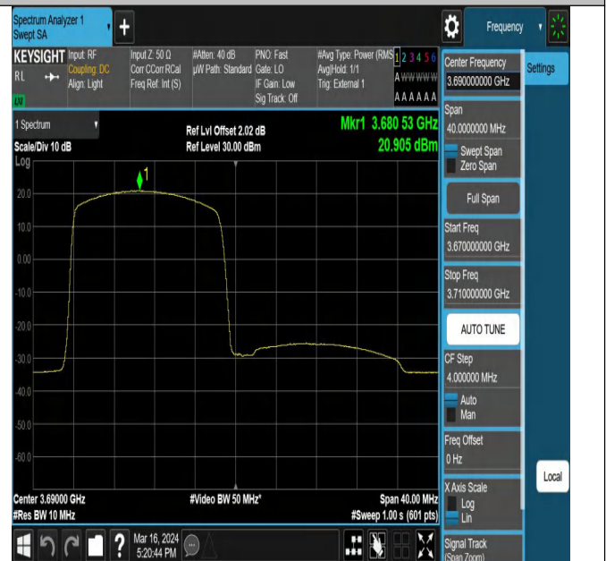
43(3600-3700)-20MHz-16QAM-44490-1RB#0-PASS
