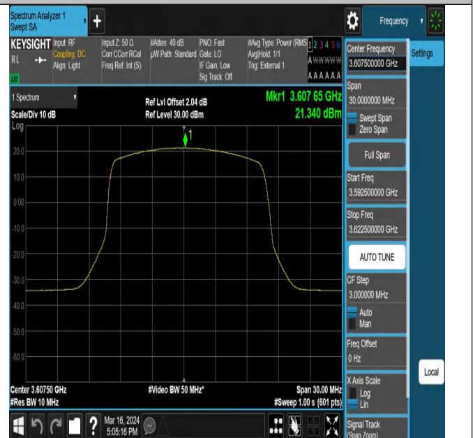
43(3600-3700)-15MHz-16QAM-43665-1RB#38-PASS
