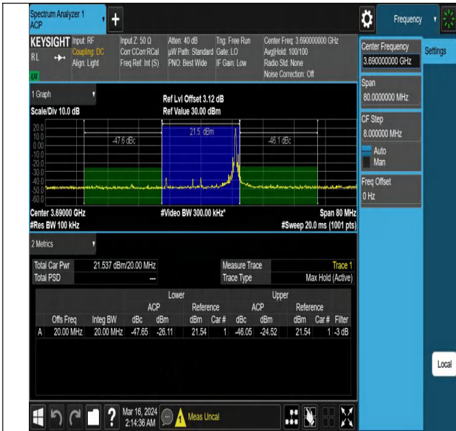
43(3600-3700)-20MHz-QPSK-44490-1RB#99-PASS
