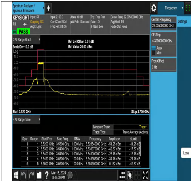
Band42_10MHz_QPSK_43140_50RB#0
