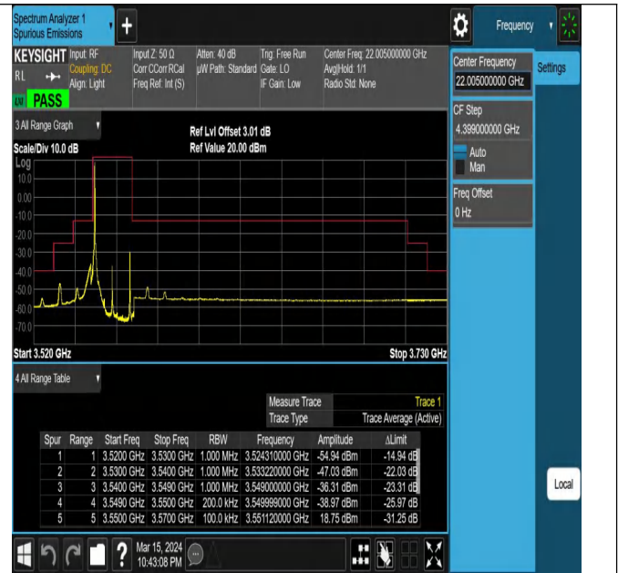
Band42_20MHz_QPSK_43190_1RB#0
