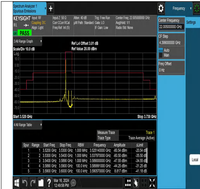
Band42_10MHz_QPSK_43540_1RB#0
