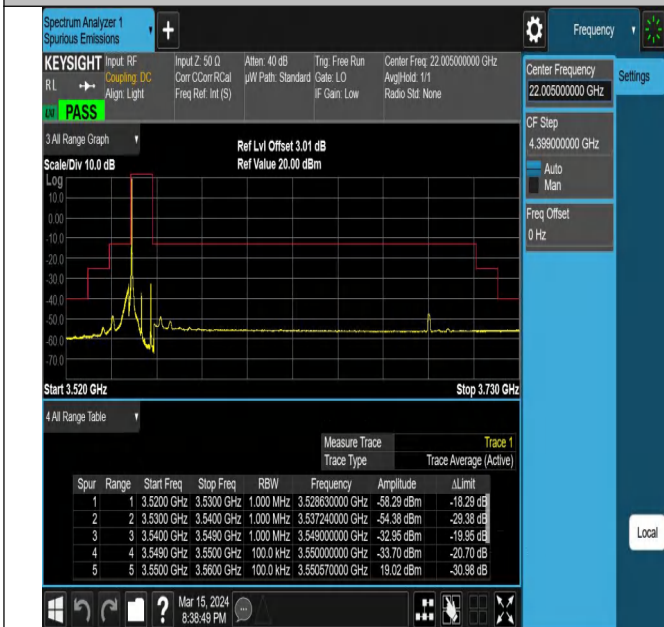
Band42_10MHz_QPSK_43140_1RB#0
