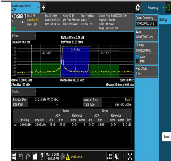
42(3550-3600)-20MHz-QPSK-43190-1RB#0-PASS
