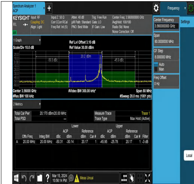
42(3550-3600)-20MHz-16QAM-43190-1RB#99-PASS
